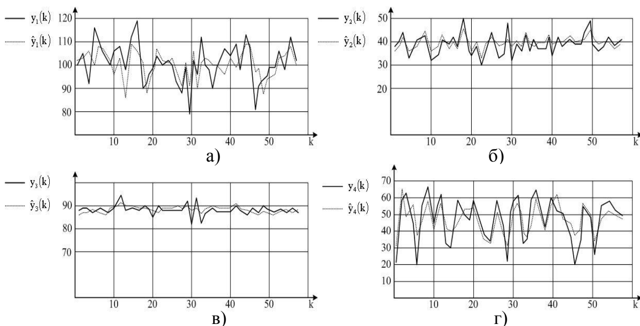
Рисунок 3 – Зміни реальної ( y ) та модельної ( \hat{y} ) вихідних змінних дифузійного відділення - температури сокостружечної суміші, для моделей (5)-(8): а) в 1-й зоні ДА ; б) 2-й зоні ДА; в) в 3-й зоні ДА; г) в 4-й зоні ДА
