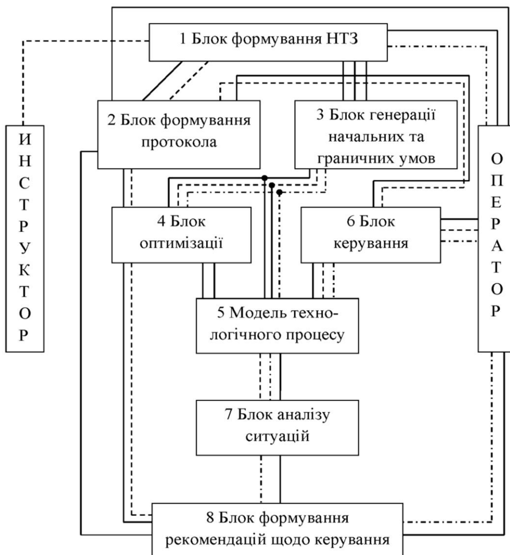
Рисунок 5 – Структура імітаційної навчальної моделі
