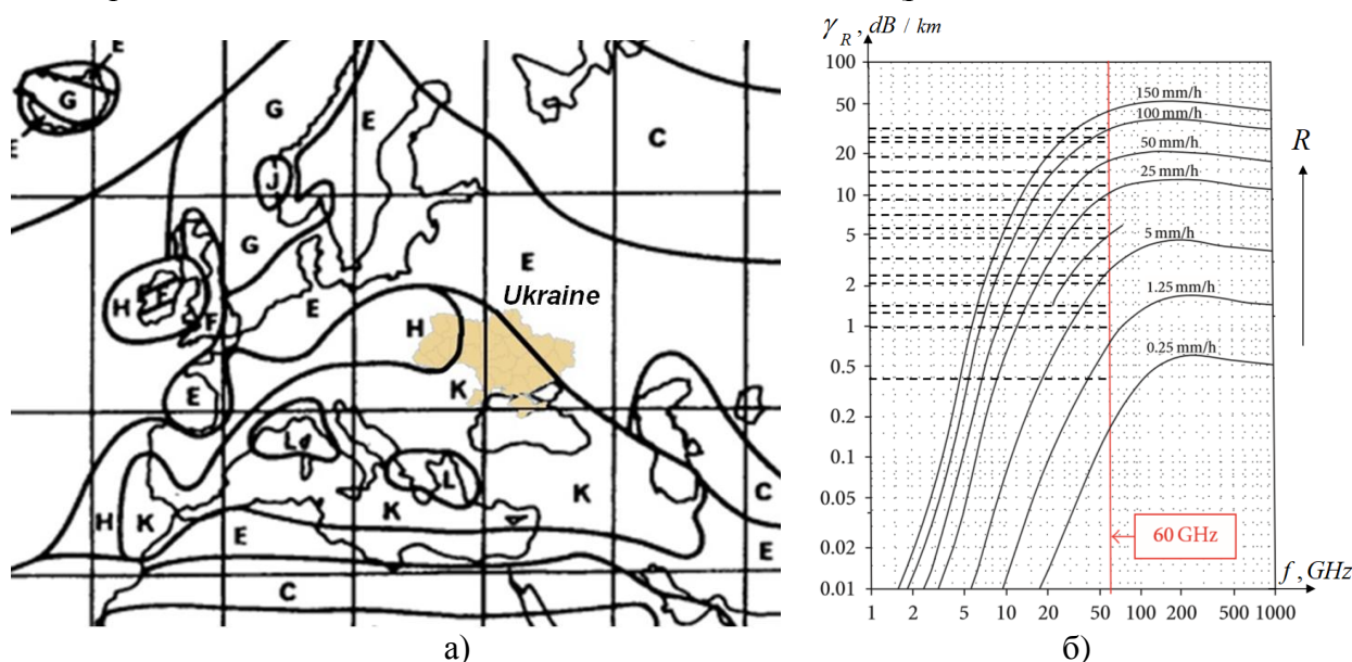
Рис. 3. Расположение Украины в трех климатических зонах ITU (а) и зависимость погонного затухания \gamma_R от частоты сигнала и интенсивности осадков R (б)
