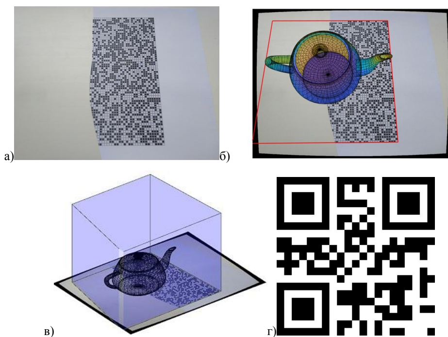
Рис. 9. Приклад використання мозаїчного стохастичного AR-маркера: а) вихідне зображення; б) точний метод проєктування віртуального 3d об'єкту в область маркера; в) спрощений метод проєктування віртуального 3d об'єкту в область маркера; г) декодоване зображення-повідомлення
