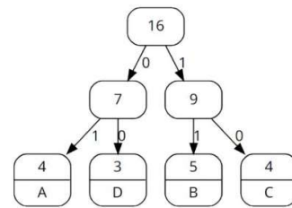
Рис. 2. Приклад діаграми Хаффмана
