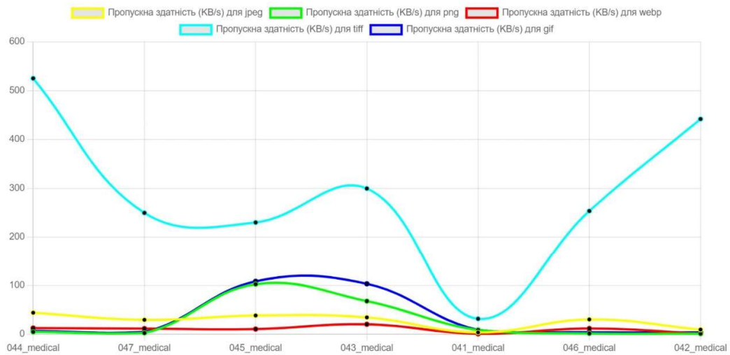
Рис. 9. Графік пропускної здатності для медичних зображень
