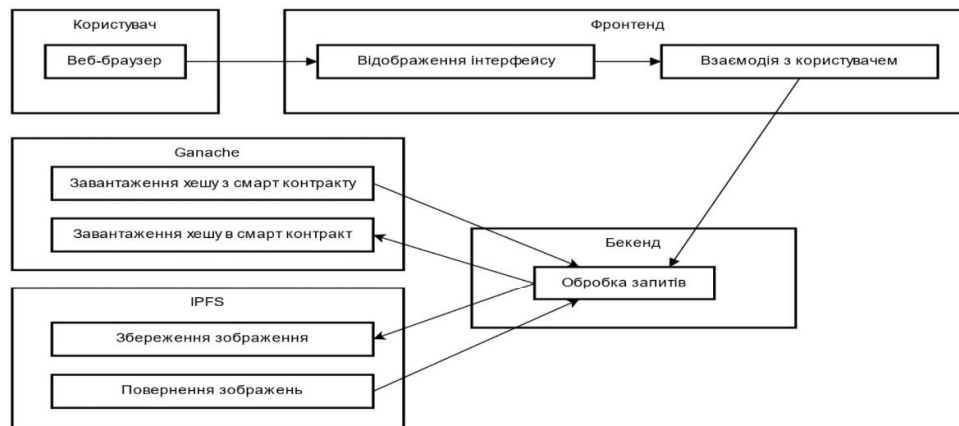
Рис. 3. Архітектура пропонованого застосунку для аналізу.
