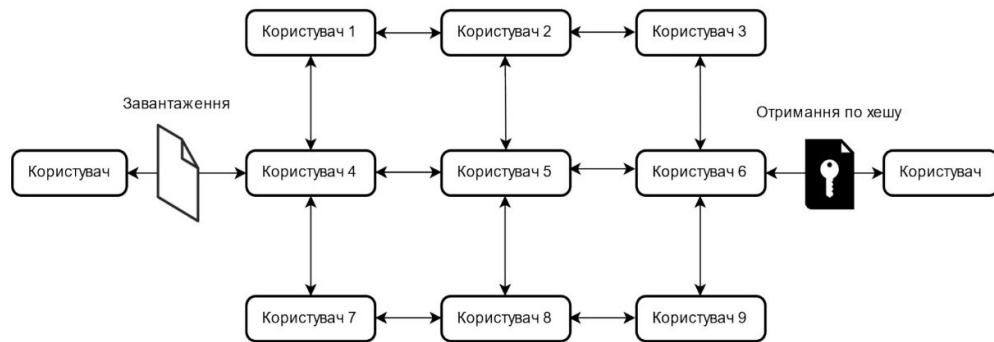
Рис. 1. Архітектура сучасних блокчейн сховищ
