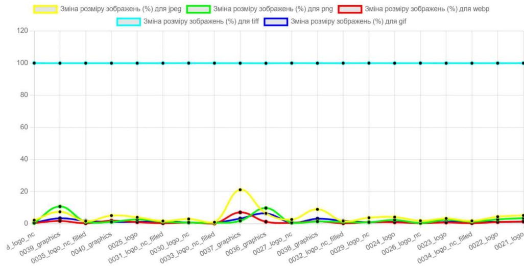
Рис. 10. Графік зміни розміру графічних зображень і логотипів
