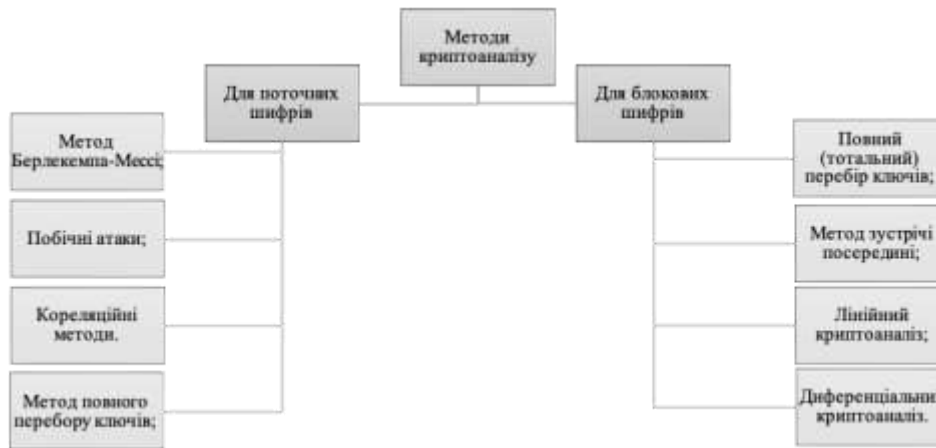
Рисунок 1 – Методи криптоаналізу.
