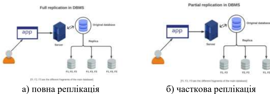
Рисунок 1 – Схема реплікації
