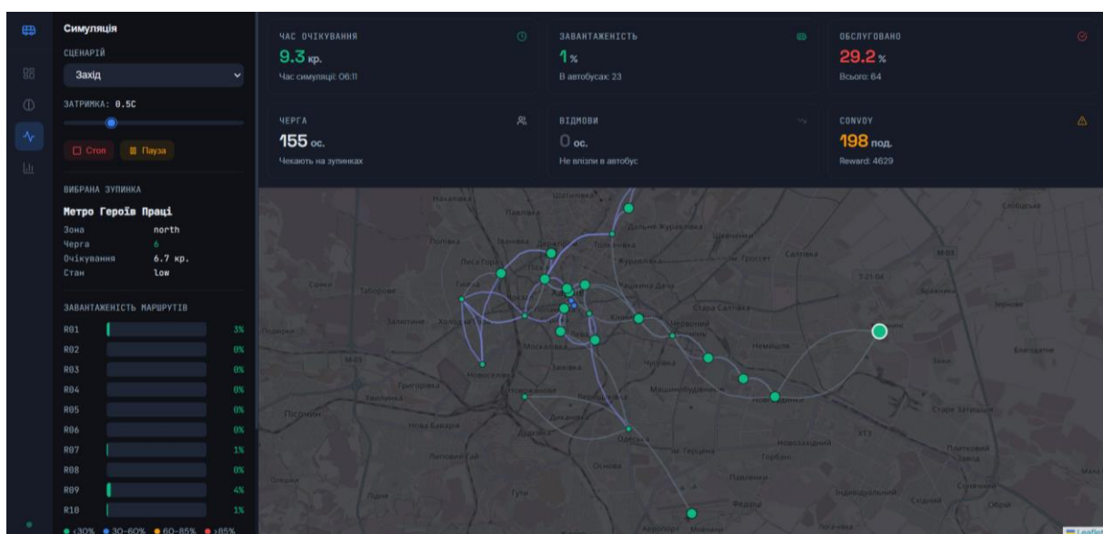
Рисунок А.8 – Сценарій mass_event: масовий захід з підвищеним навантаженням
