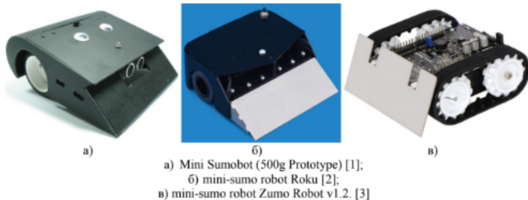
Рисунок 1 – Загальний вид мобільних роботів класу Mini Sumo для Robot Battle
