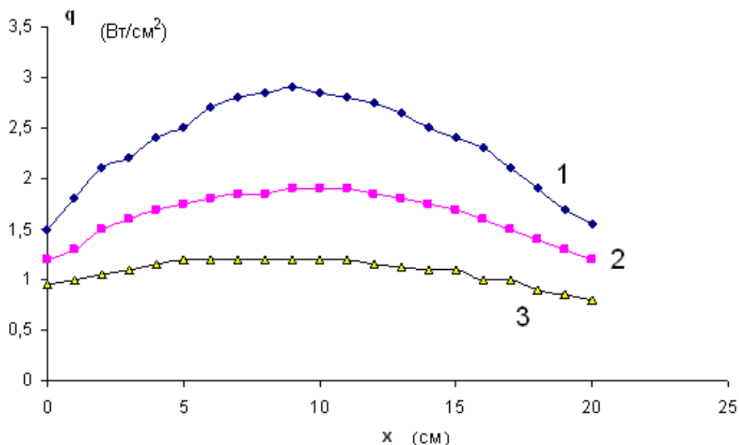
Рис.1. Распределения плотности энергии нагревателя для дистанции, 1 – 20 (см), 2 – 30 (см), 3 – 40 (см).
