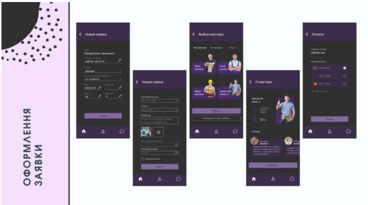
Рисунок А.18 – Екранні форми оформлення заявки мобільного додатку «Мій майстер»
