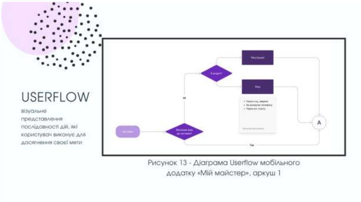
Рисунок А.12 – Userflow мобільного додатку «Мій майстер»
