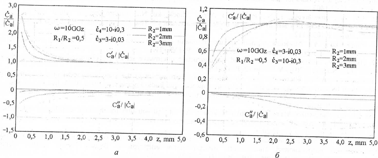
Рис. 4. Относительное изменение емкости апертуры при а) |\dot{\epsilon}_4| > |\dot{\epsilon}_3| ; б) |\dot{\epsilon}_3| > |\dot{\epsilon}_4|
