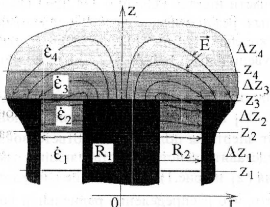
Рис. 1. Геометрическая схема рабочей области коаксиального сенсора
