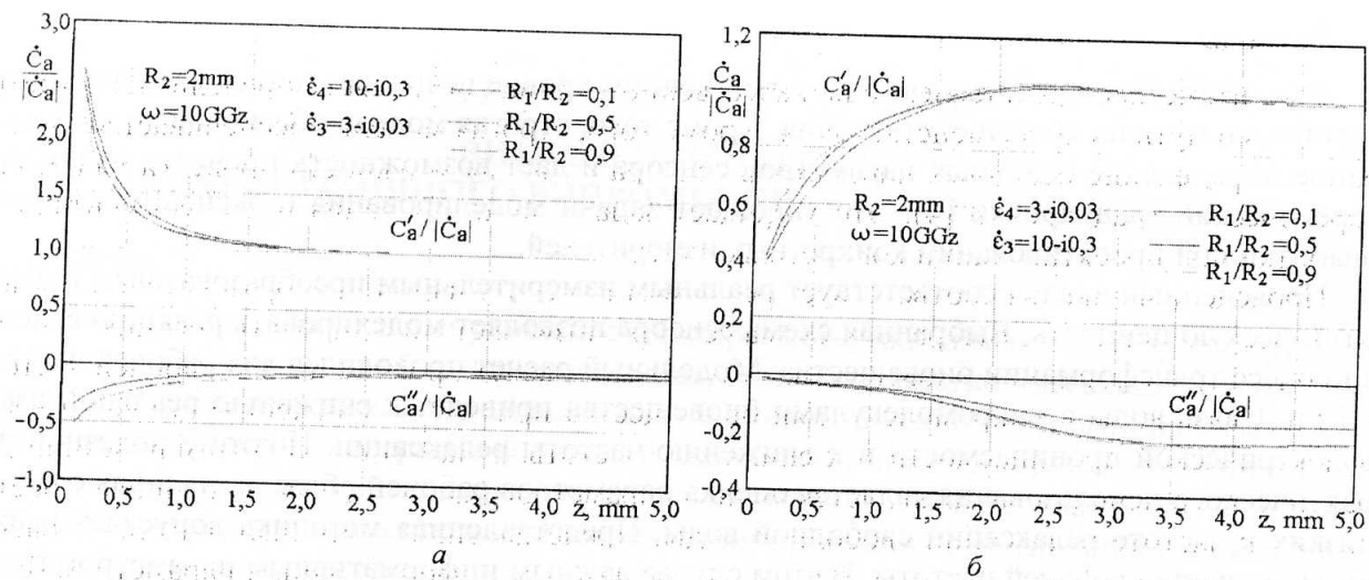
Рис. 3. Относительное изменение емкости апертуры при а) |\dot{\epsilon}_4| > |\dot{\epsilon}_3| ; б) |\dot{\epsilon}_3| > |\dot{\epsilon}_4|
