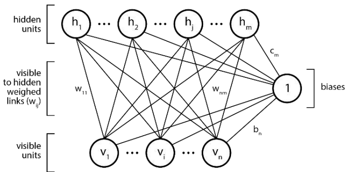
Рис. 1. Структура Обмеженої машини Больцмана.
