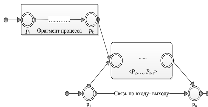
Рис. 4 – Взаимодействие конструкции неявного выбора с другими фрагментами бизнес-процесса: связь по входу в \langle P_2, \dots, P_{n-1} \rangle
