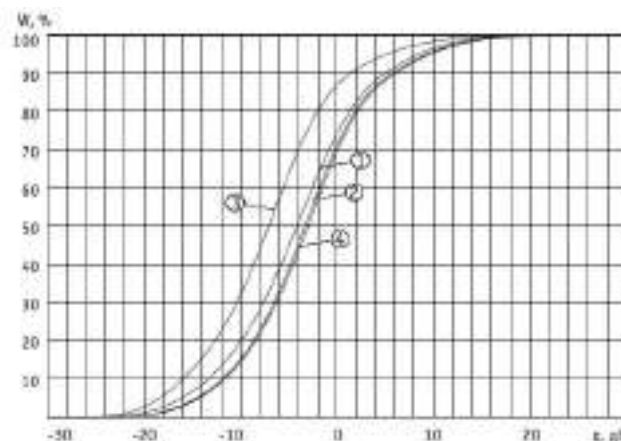
Рис.1 Залежність словесної розбірливості W від інтегрального відношення сигнал/шум q в смузі частот 175...5600 Гц: 1- "білий" шум; 2 – "рожевий" шум; 3 – "коричневий" шум; 4 – мовоподібний шум
