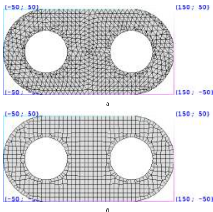
Рис. 10. Приклади результатів алгоритму для області, заданій формулою (1): а – трикутники, б – чотирикутники
