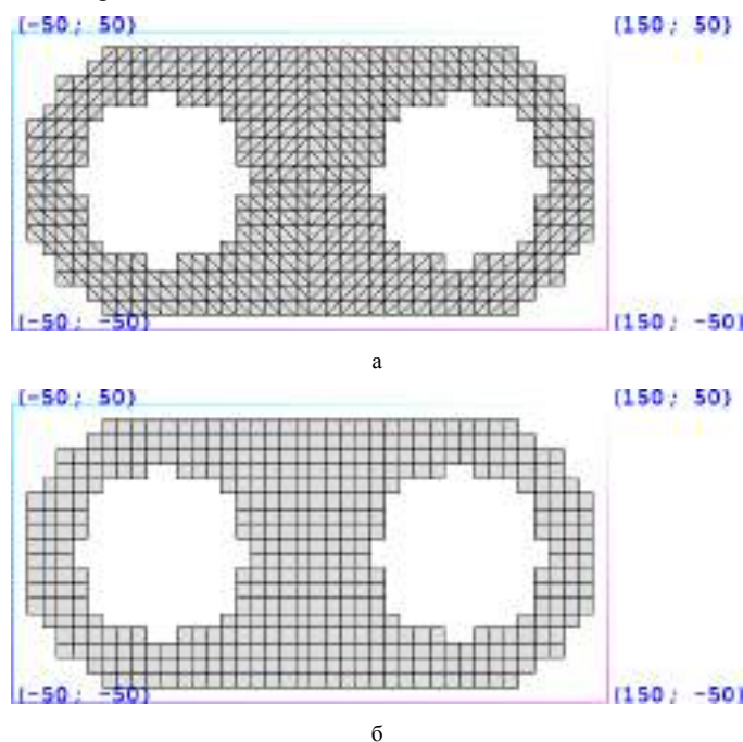
Рис. 9. Приклади виконання першого кроку алгоритму для області, заданій формулою (1), при рівномірній структурованій фоновій дискретній моделі: а – трикутники, б – чотирикутники
