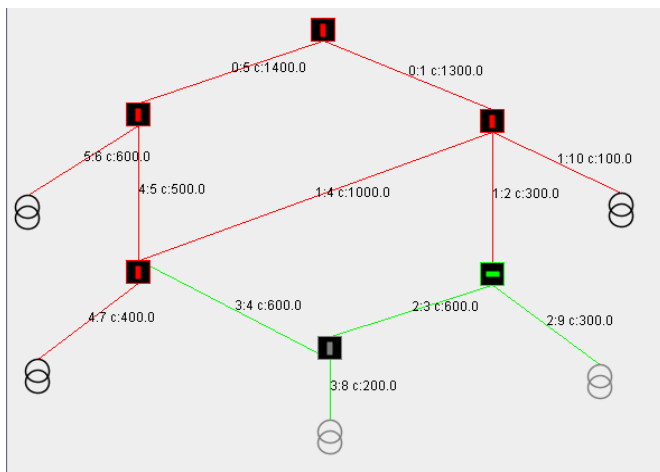
Рис.19. Вигляд мережі після перемикання
