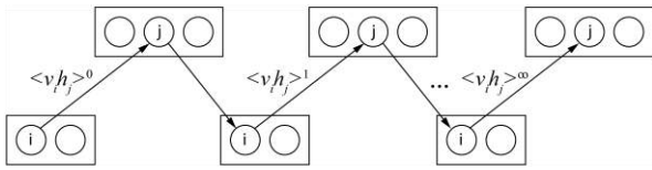
Рис. 2. Алгоритм CD-k при k \rightarrow \infty
