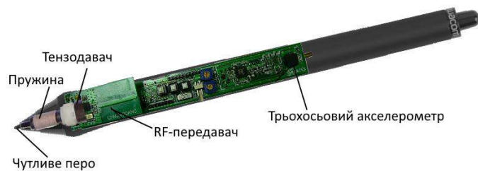
Fig. 3. Пристрій графічного цифрового пера з вбудованим 3D-мікроакселерометром для проведення діагностичного тесту
