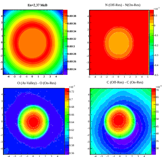
Рис. 2. Результати моделювання отримання радіографічного зображення при розташуванні об'єкту з матеріалу 1 у ґрунті
