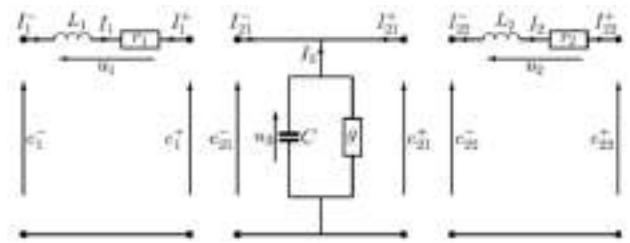
Рис. 3. Четырехполосники, реализующие звенья декомпозиции \Phi = \Phi_1 \otimes \Phi_{21} \otimes \Phi_{22} .
