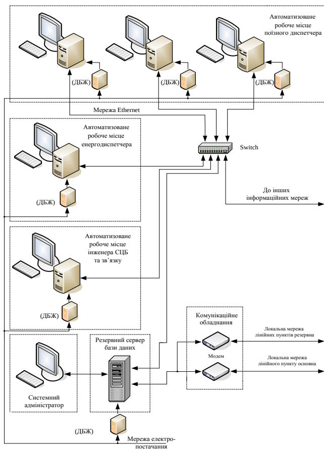
Рис. 2. Структурна схема «ДЦ Каскад»
