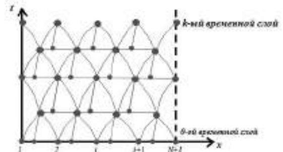
Рис. 1 – Сітка для розрахунку параметрів газового потоку.
