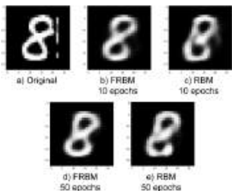
Рис. 7. Результати відтворення зразка «8» із артефактом після усього 10 навчальних епох: а) оригінальний зразок; б) відтворення нечіткою ОМБ після 10 епох; с) відтворення класичною ОМБ після 10 епох; д) відтворення нечіткою ОМБ після 50 епох; е) відтворення класичною ОМБ після 50 епох.
