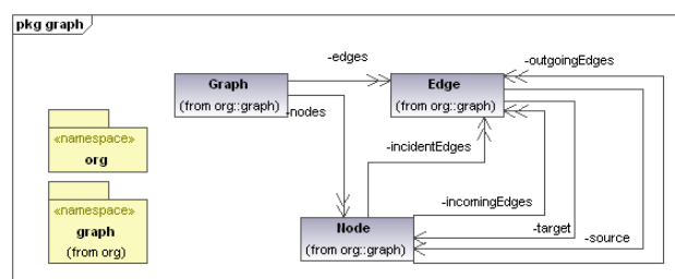
Рис.13. UML діаграма пакету org.graph
