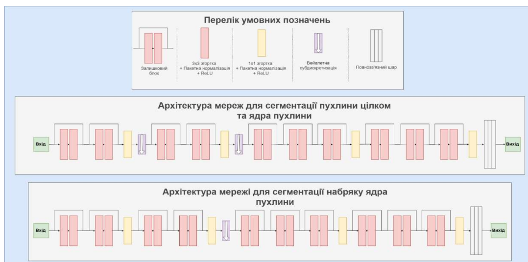
Рис. 2. Архітектура нейронних мереж для сегментації пухлин головного мозку
