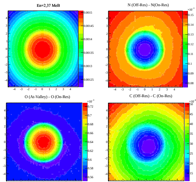
Рис. 3. Результати моделювання отримання радіографічного зображення при розташуванні об'єкту з матеріалу 2 у ґрунті
