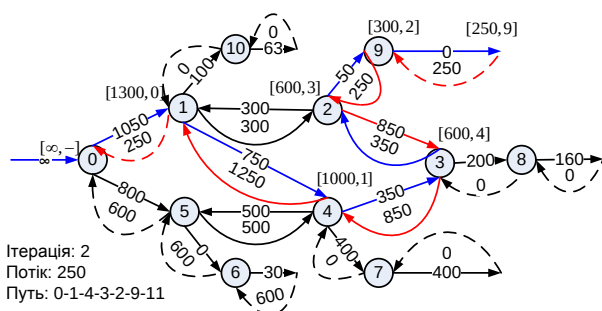
Рис.8. Мережа після другої ітерації алгоритму
