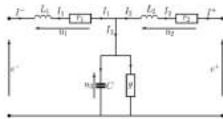
Рис. 2. Четырехполюсный фильтр.
