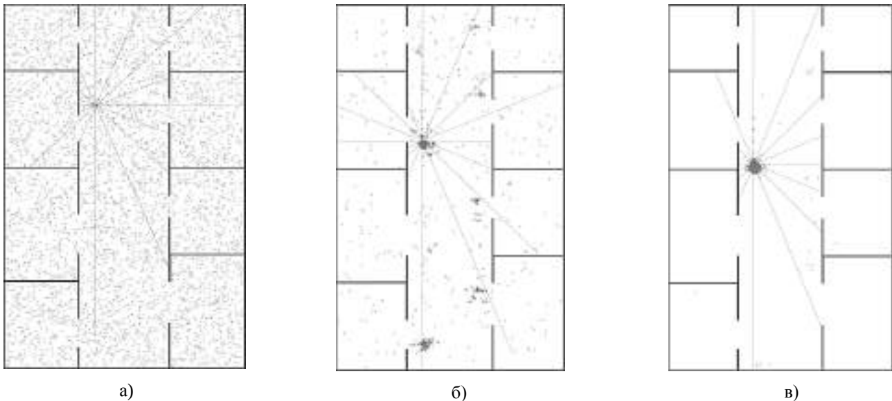
Рис. 7. Результати моделювання визначення місця розташування автономного робота в будівлі: а) робот генерує безліч припущень про своє місцезнаходження, б) формуються кластери з найбільш високими можливостями, в) робот визначив своє місце розташування
