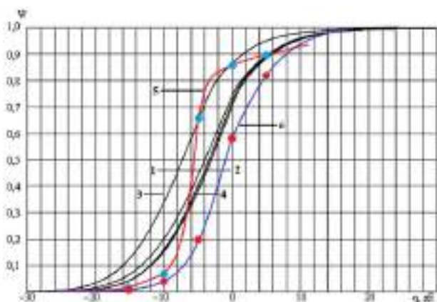
Рис.2 Залежність словесної розбірливості W від інтегрального відношення сигнал/завада q : 1 – "білий" шум; 2 – "рожевий" шум; 3 – "коричневий" шум; 4 – мовоподібний шум; 5 – реальна мовоподібна завада сформована генератором ОССА-1 до модернізації; 6 – реальна мовоподібна завада сформована генератором ОССА-1 після модернізації
