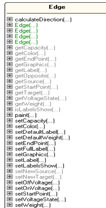
Рис.15. Клас Edge
