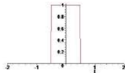
Рис. 1 В-сплайн B_{0,h}(t) .
