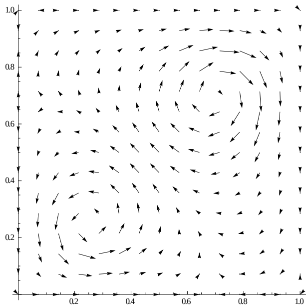
Рис. 2. Поле швидкостей.
