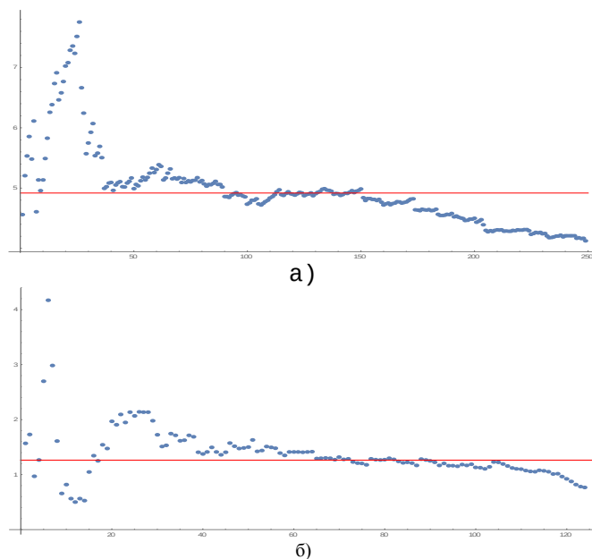
Рис.2 – Оцінювання хвостового індексу для значення лептону рТ.
