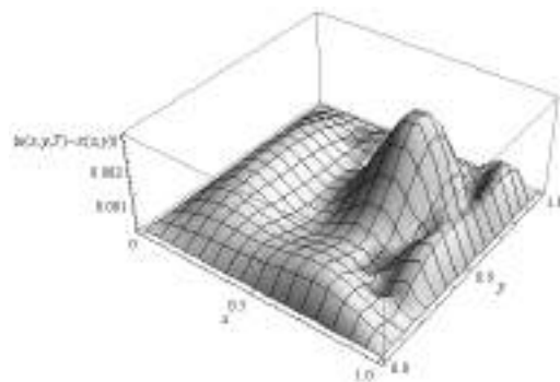
Рис. 8. Відхилення |u(x, y, T) - z(x, y)|
