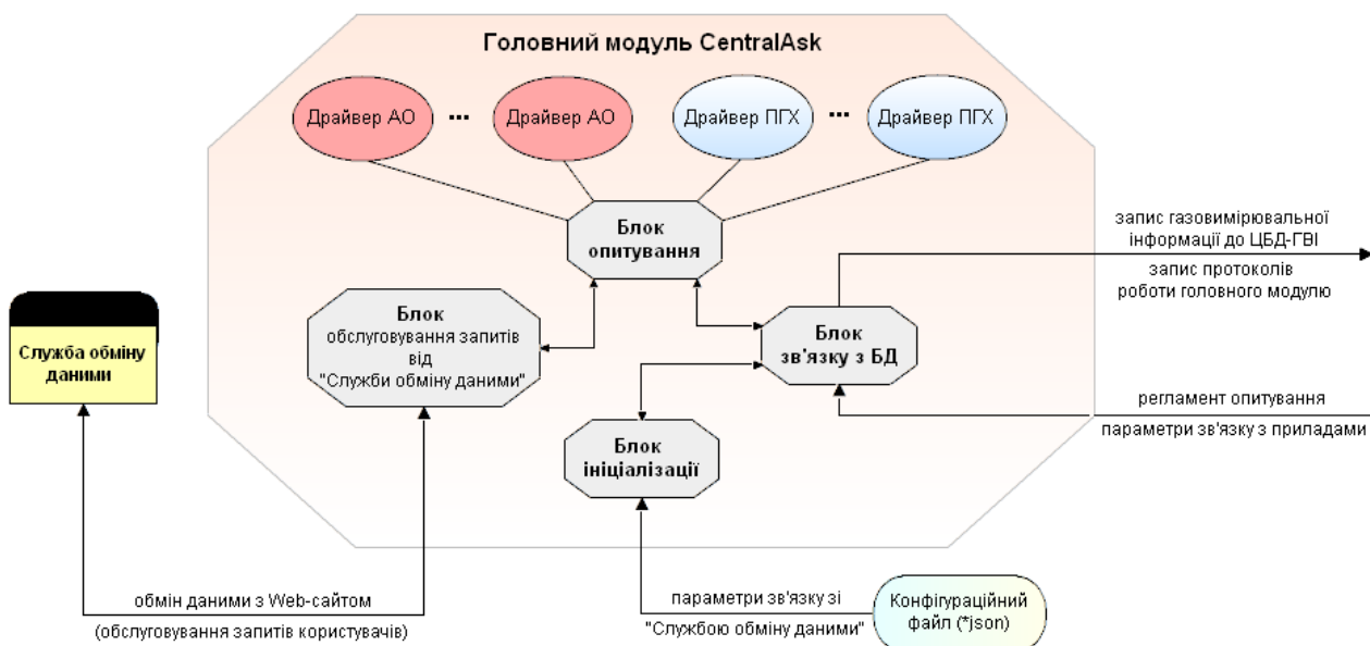
Рис. 1. Структурна схема головного модуля ПК CentralAsk.
