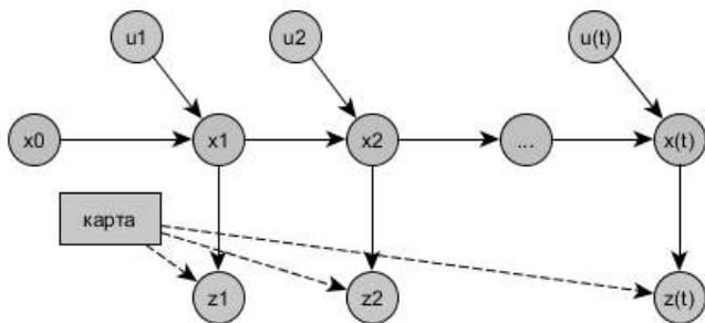
Рис. 4. Графічний вигляд представлення процесу руху робота в просторі
