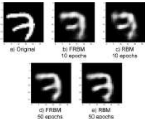
Рис. 6. Результати відтворення зразка цифри «7»: а) оригінальний зразок; б) відтворення нечіткою ОМБ після 10 епох; с) відтворення класичною ОМБ після 10 епох; д) відтворення нечіткою ОМБ після 50 епох; е) відтворення класичною ОМБ після 50 епох.
