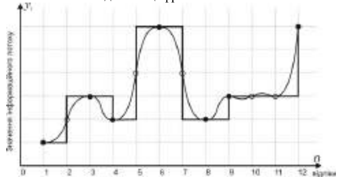
Рис. 1. Цифровий сигнал.
