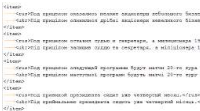
Рис. 4 – Зразок паралельного корпусу
