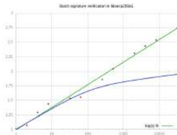
Рис. 2. График сравнения ECDSA и подписи Шнорра.
