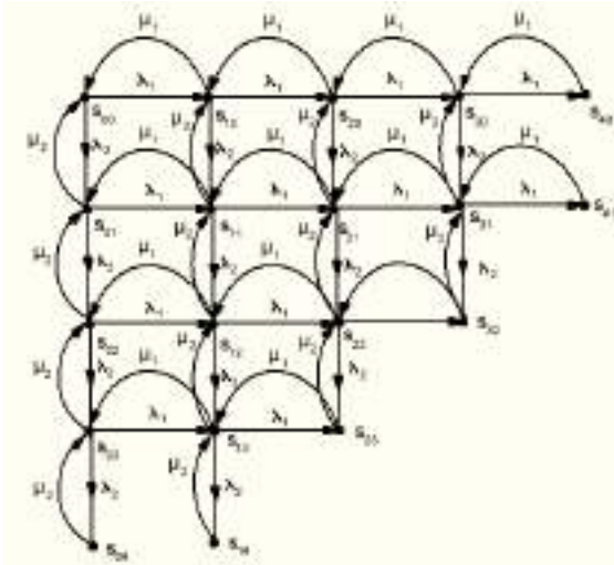
Рис. 1. Граф станів і переходів досліджуваної системи у випадку n = 2, N = 3
