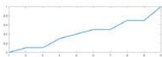
Рис. 5 Первая производная сплайна
