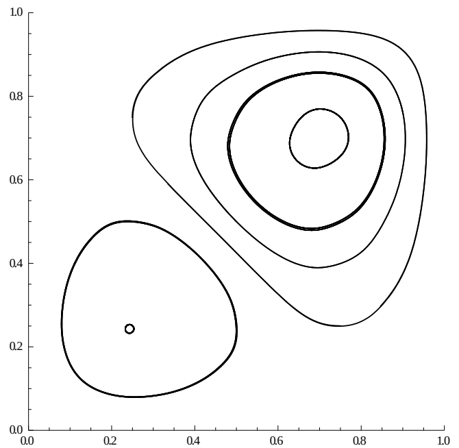
Рис. 3. Фазові траєкторії.
