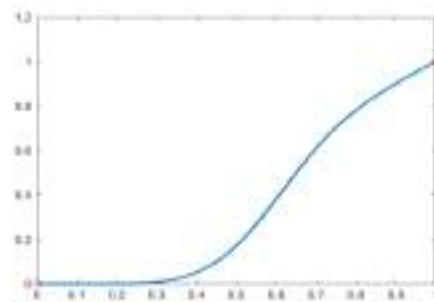
Рис. 4 Описание IRT функции тестирования параболическим сплайном
