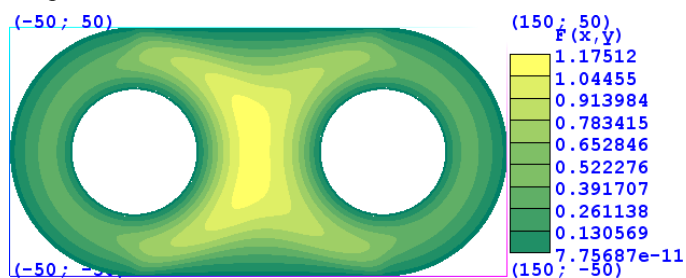
Рис. 7. Розподіл значень функції (1) у середині області
