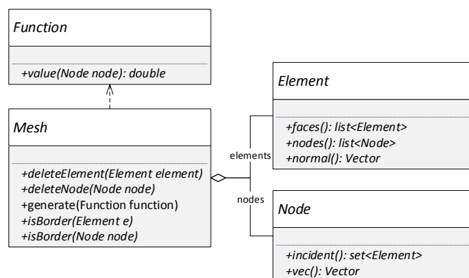
Рис. 13. Діаграма класів
