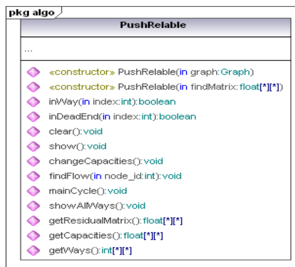
Рис.11. Клас PushRelabel
