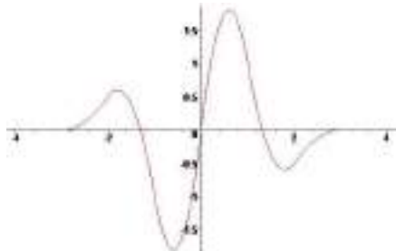
Рис. 3 В-сплайн B_{5,h}^{(3)}(t) .
