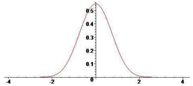
Рис. 2 В-сплайн B_{5,h}(t) .
