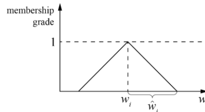
Рис. 3. Симетричне трикутне нечітке число.
