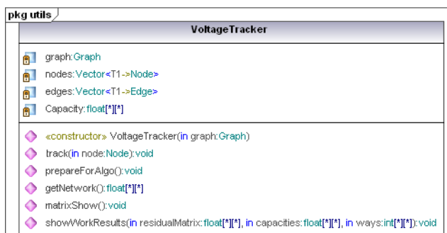
Рис.12. Клас VoltageTracker
