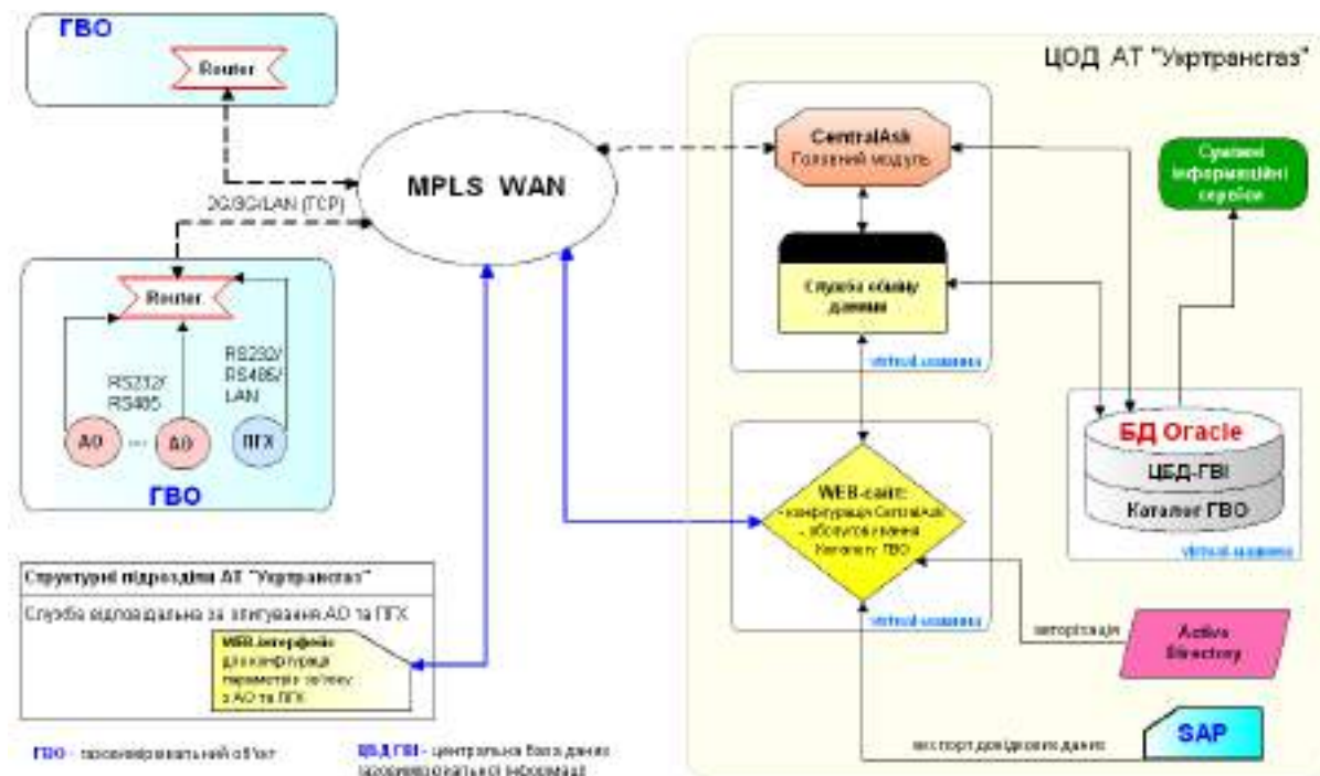
Рис. 2. Структурна схема ПК CentralAsk.
