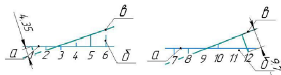
Рис. 9. Відхилення від прямолінійності для площини IV
