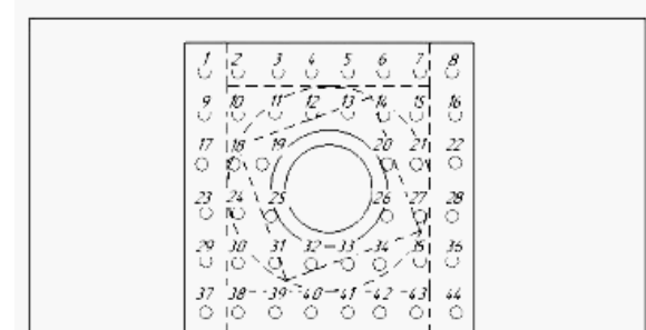
Рис. 10. Схема вимірювання паралельності торцевої поверхні повернутого паралелепіпеда
