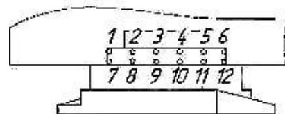
Рис. 5. Схема вимірювань площинності торцевої поверхні повернутого паралелепіпеда
