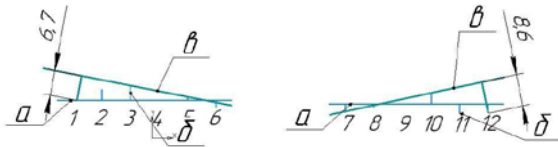
Рис. 7. Відхилення від прямолінійності для площини II
