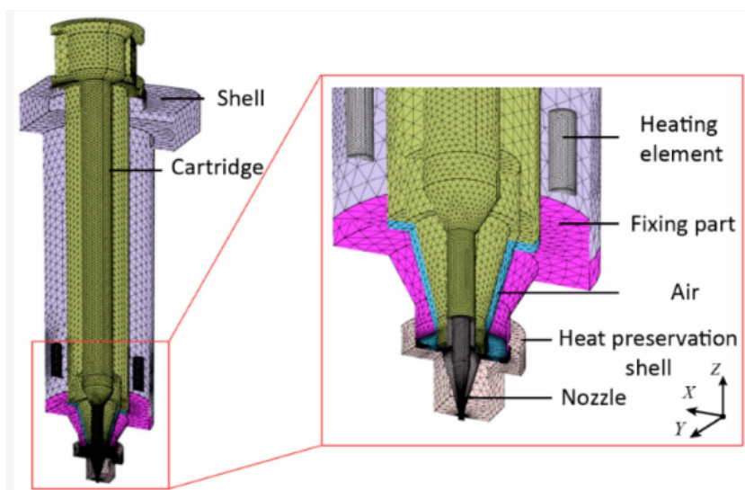
Рисунок 2 – Спрощення моделі FEM екструдера
