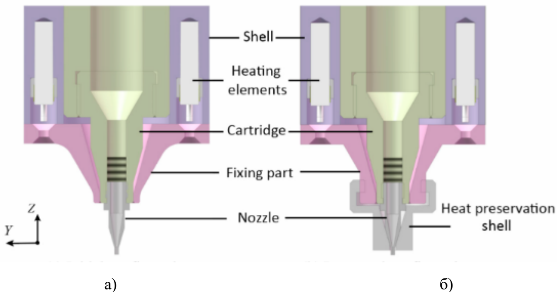
Рисунок 1 – Покращена конфігурація на основі вихідної друкуючої голівки
