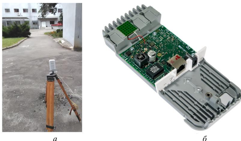
Рис. 8. Экспериментальная линия связи ( а ) диапазона 60 ГГц на основе радиомодемов MikroTik Wireless Wire ( б )
