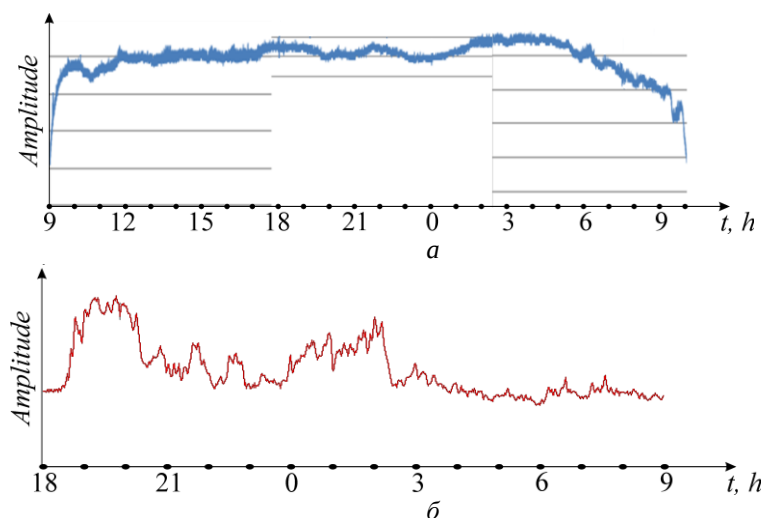
Рис. 9. Фрагменты записи изменения радиояростной температуры неба в 3 см ДВ (а – апрель 2017) и 3 мм ДВ (б – май) при прохождении двух весенних атмосферных фронтов над измерительным пунктом в течение 25 и 16 часов соответственно
