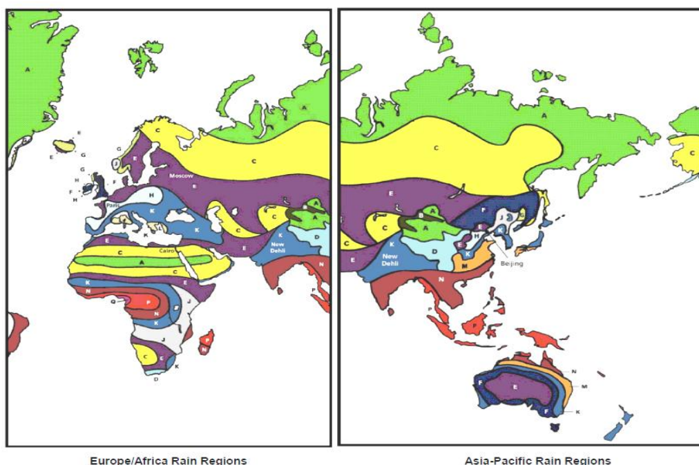
Рис. 3. Укрупненная карта климатических зон по ИТУ [2]
