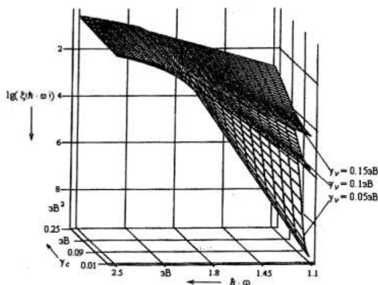
Рис. 4. Спектральные зависимости нормированной обобщенной функции распределения плотности состояний
