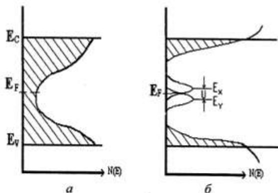
Рис. 1. Различные виды плотности состояний в электронных в аморфных полупроводниках: а – модель Козна – Фриче – Овчинского; б – модель Мота – Дэвиса
