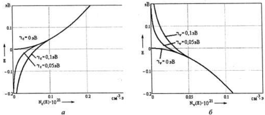
Рис. 2. Зависимости плотности состояний для: а – зоны проводимости и б – валентной зоны
