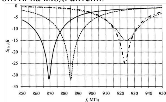
Рис. 6 - - - - - антена з вирізами в екрані, l_2=17 мм — антена з вирізами в екрані, l_2=17 мм та корегованою довжиною випромінювача ..... антена без вирізів в екрані, l_2=17 мм - . - антена без вирізів в екрані, l_2=15 мм
