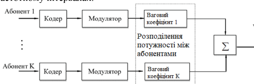
Рисунок 3 Структурна схема передачі PD-NOMA
