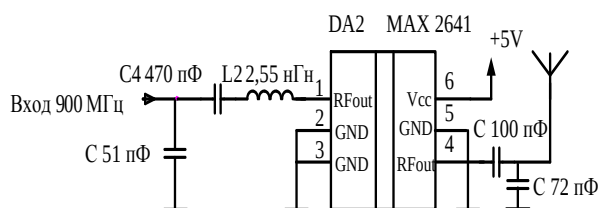
Рисунок 4 – ПП на частоту 1800 МГц
