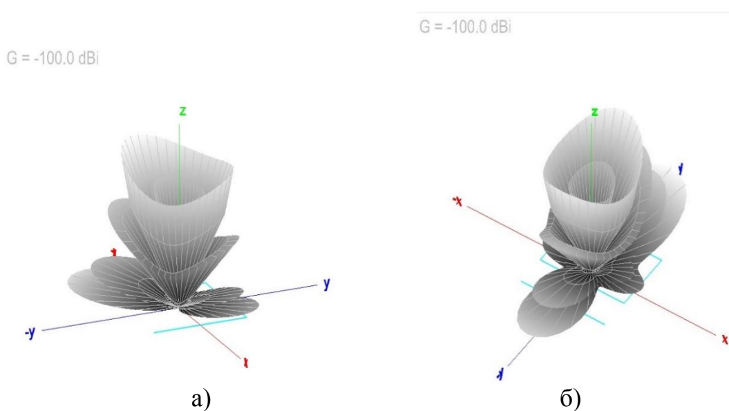
Рисунок 3 – Діаграми спрямованості антен першої (а) та другої (б) ітерації кривої Гільберта у MMANA-GAL
