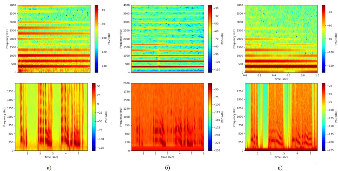
Рисунок 1 – Спектрограми сигналу
