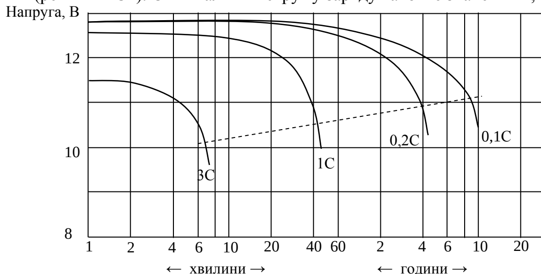
Рис. 1. Розрядні характеристики батареї EPS 1220
