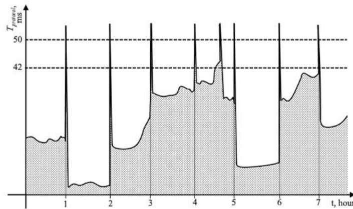
Рисунок 2 – Приклад часових затримок, які виникають при перебудові ланцюга
