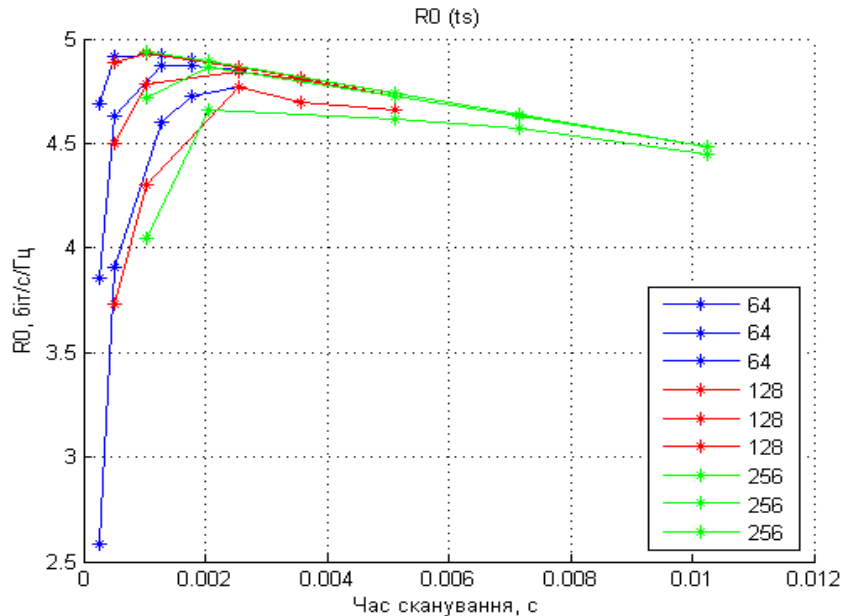
Рис. 8. Залежність нормованої досяжної пропускної здатності для вторинної мережі КР від часу сканування ( v ) при різних значеннях ВССШ та різних розмірностях ДПФ ( T = 100 мс)
