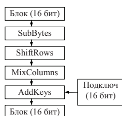
Рис. 3. Схема одного цикла SPN-шифра
