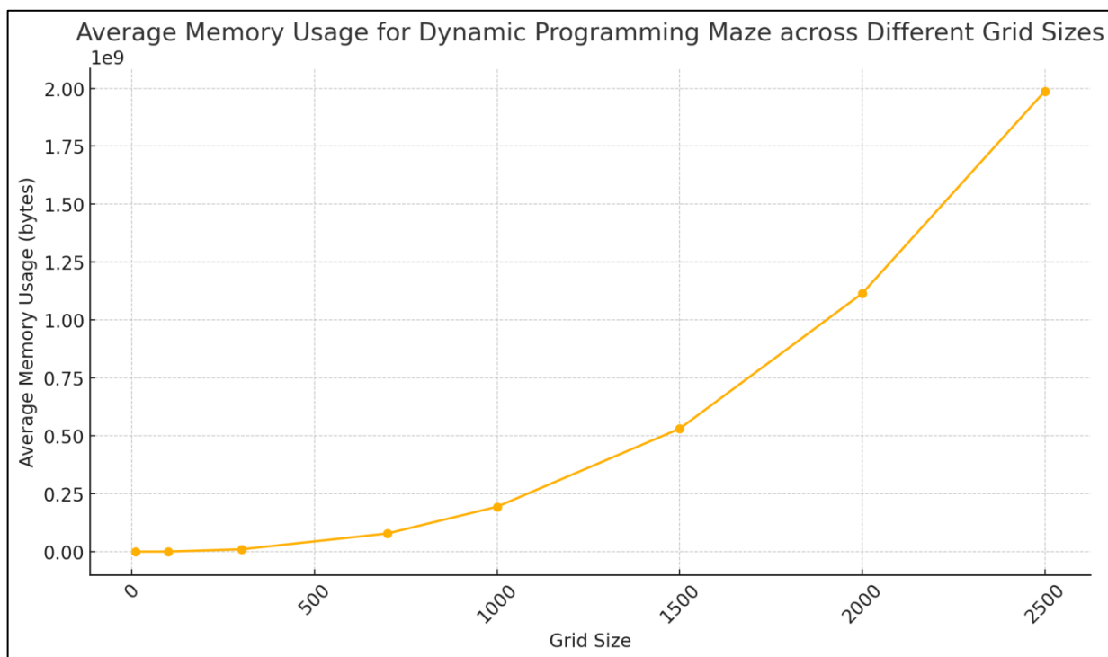
Рисунок 5.6 – Середнє значення використання пам'яті Dynamic Programming Maze (рисунок створено самостійно)
