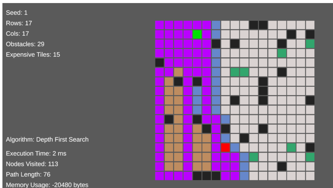
Рисунок 4.13 – Приклад роботи алгоритму DFS на сітці 17x17 тайлів (створено самотійно)
