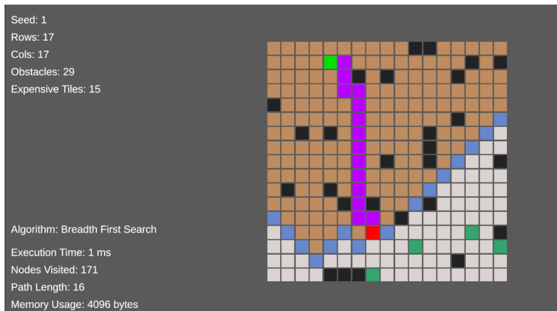
Рисунок 4.5 – Приклад роботи BFS на сітці 17x17 тайлів
