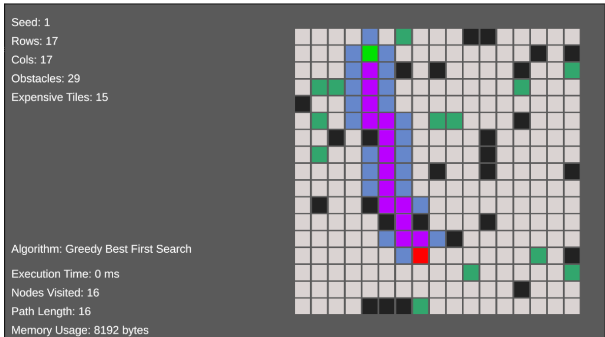
Рисунок 4.11 – Приклад роботи алгоритму Greedy Best First Search на сітці 17x17 тайлів (створено самостійно)
