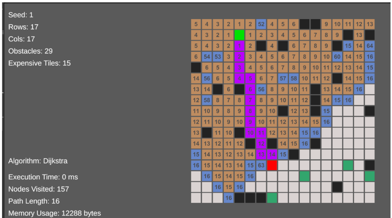
Рисунок 4.7 – Приклад роботи алгоритму Дейкстри на сітці 17x17 тайлів
