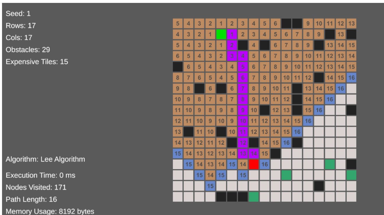
Рисунок 4.17 – Приклад роботи алгоритму Lee на сітці 17x17 тайлів (створено самотійно)
