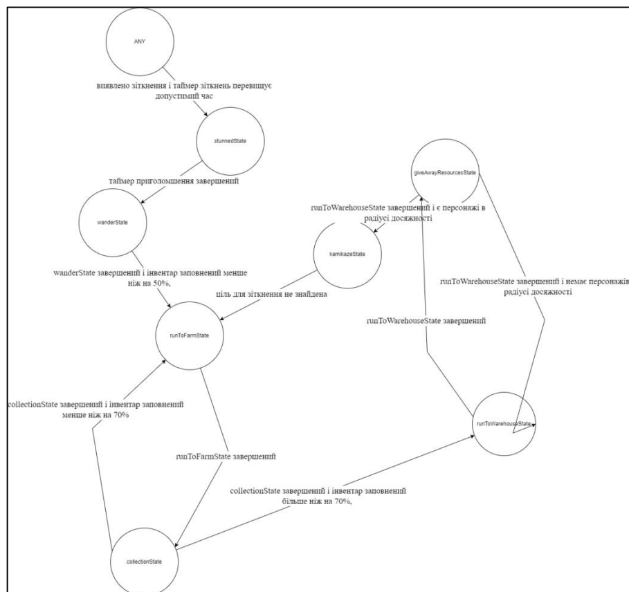
Рисунок 4.30 – Схема переходів станів у StateMachine (створено самостійно)
