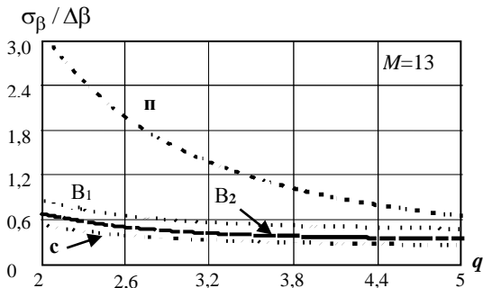
Рис. СКО измерения азимута ВО
