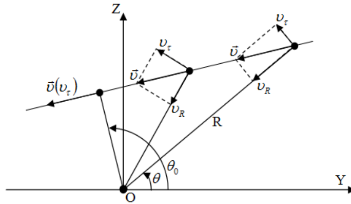
Рис. 5. Динамика изменения v_R и v_\tau для случая прямолинейного двухмерного движения объекта
