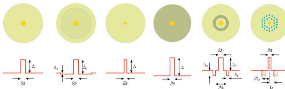
Рисунок 1 – Види поперечного перетину ОВ і їх профілі показників заломлення
