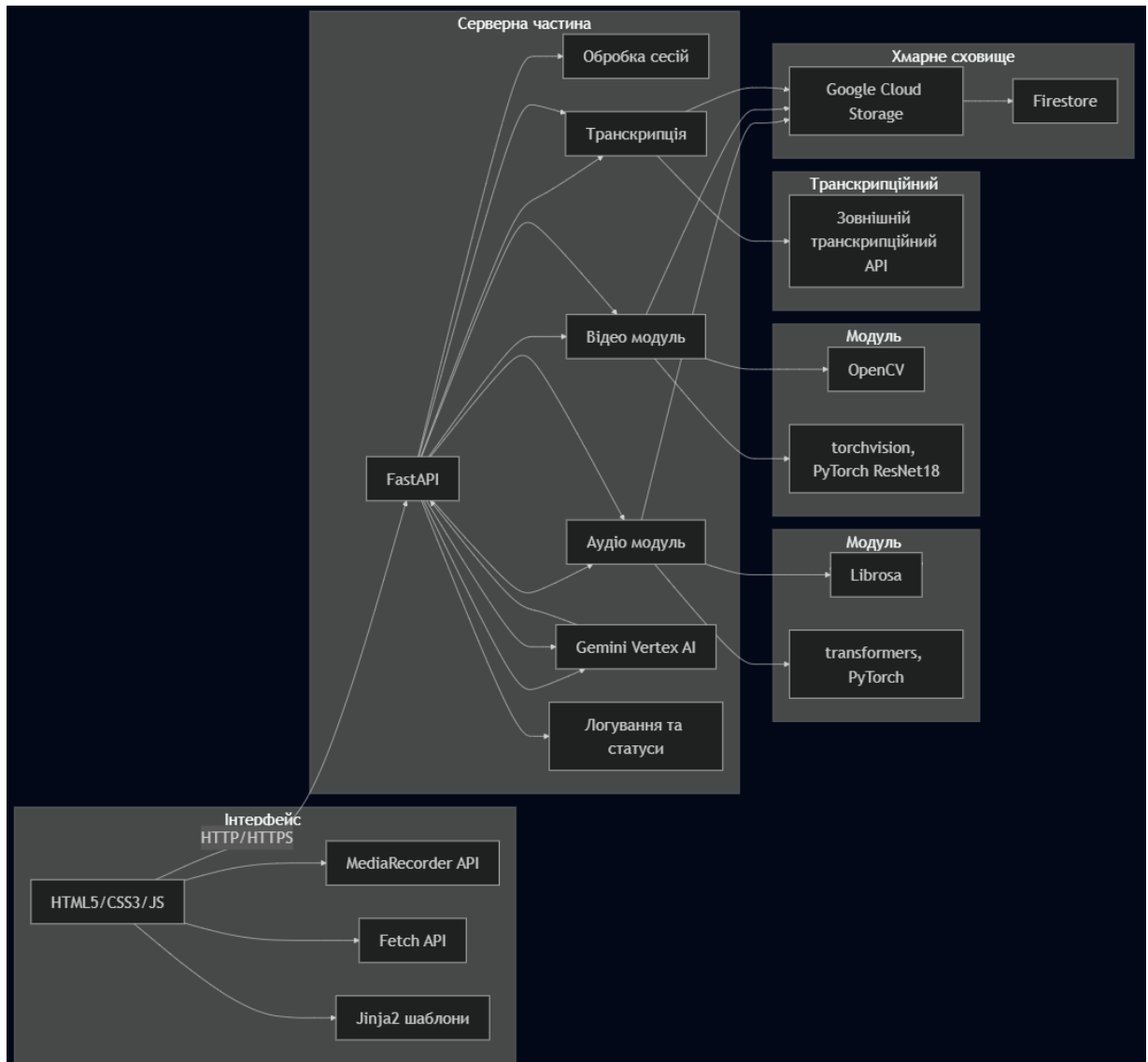
Рисунок Б.1 – Діаграма загальної архітектури вебзастосунку
