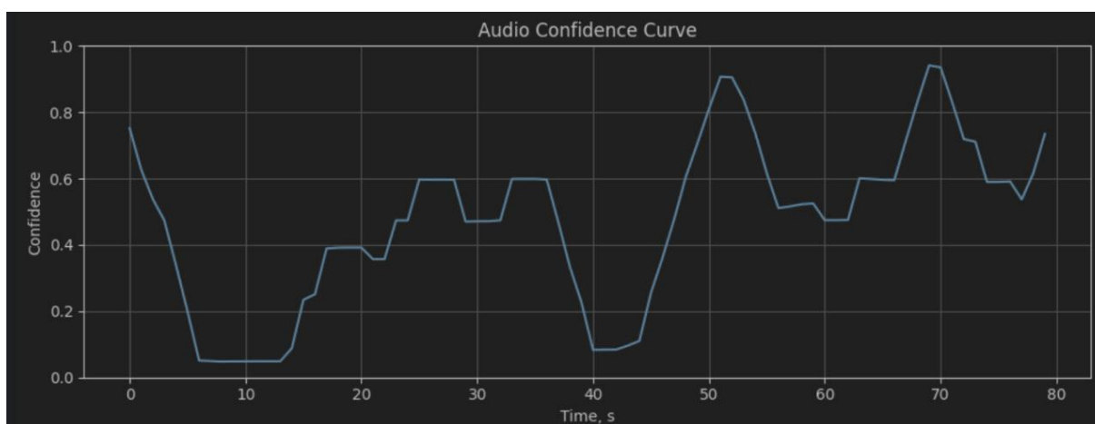
Рисунок А.2 – Результати аудіоаналізу інтерв'ю, де кандидат відчував невпевненість на середині відповіді
