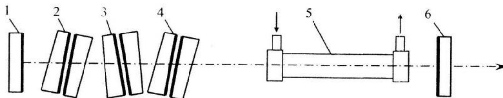
1,6 – зеркала резонатора; 2,3,4 – интерферометры; 5 – кювета с красителем
