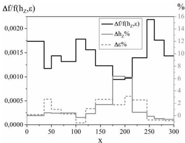
Рис. 3. Измеряемый общий профиль сигналов \Delta f/f(h_z, \epsilon) и восстановленные заданные виртуальные профили \epsilon(x) и \Delta h_z(x) в виде их процентного отклонения.
