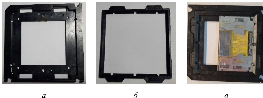
Рис. 3. Процес встановлення гнучкого надтонкого Al-Pi мікрокабелю у составну рамку TAB-70022 для фіксації та позиціонування: а – нижня рамка-основа; б – верхня рамка для кріплення мікрокабелю; в – составна рамка TAB-70022 у зборі з мікрокабелем
