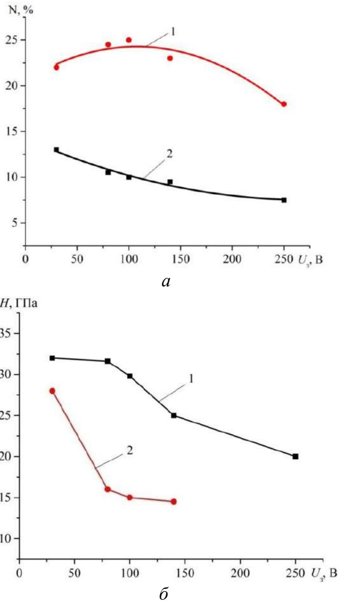
Рис. 1 – Вплив зміни потенціалу зсуву U_s на кількість азоту та твердість покриття TiNbN/CrN при тиску p = 8 \cdot 10^{-4} Торр (2) та p = 4 \cdot 10^{-3} Торр (1)
