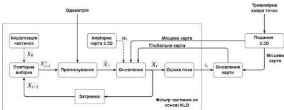
Рис. 6. Діаграма фільтра частинок на основі KLD
