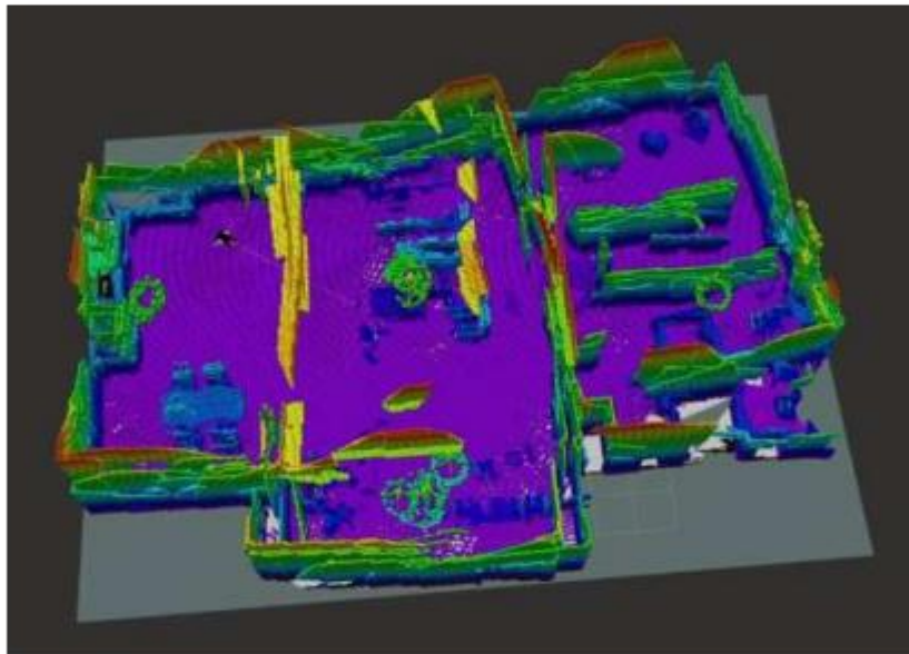
Рис. 13. Отримана 2,5D-карта висот
