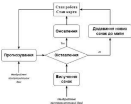
Рис. 1. Блок-діаграма процесу EKF-SLAM
