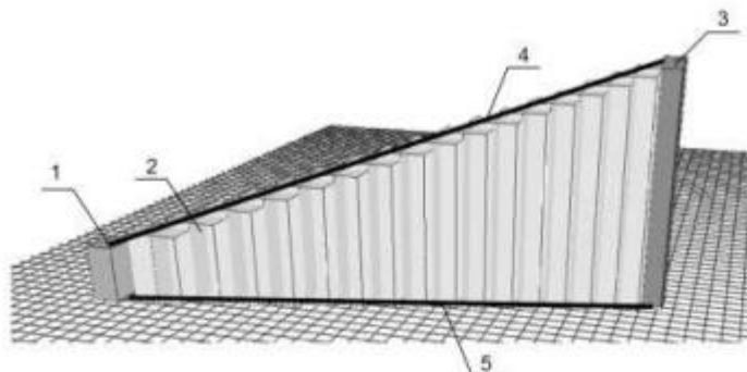
Рис. 4. Трасування ліній для одного вимірюваного висотного вокселя [19]
