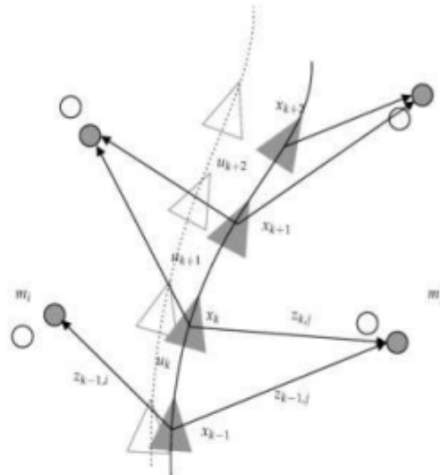
Рис. 2. Ілюстрація процесу SLAM та позначки [4]
