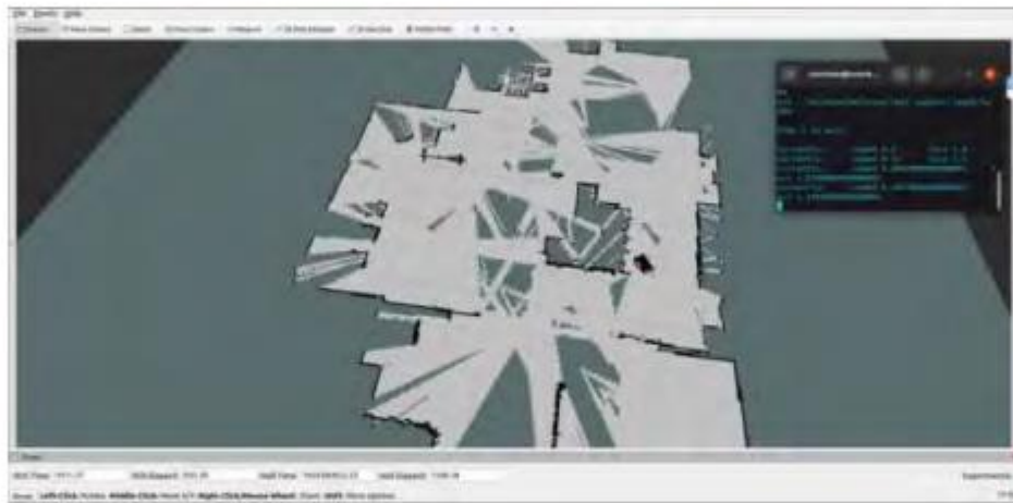
Рис. 10. Процес симуляції моделювання 2D-картографування
