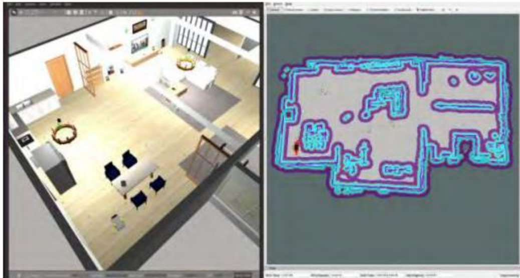
Рис. 14. Візуалізація карт вартості планування шляху
