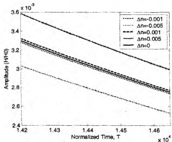
Рис. 7. Временная динамика преобразованного полного поля после серии из N импульсов
