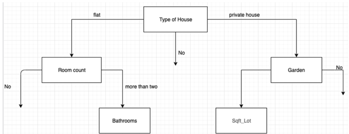
Рисунок 1 – Приклад блок-схеми реалізації алгоритму дерева рішень
