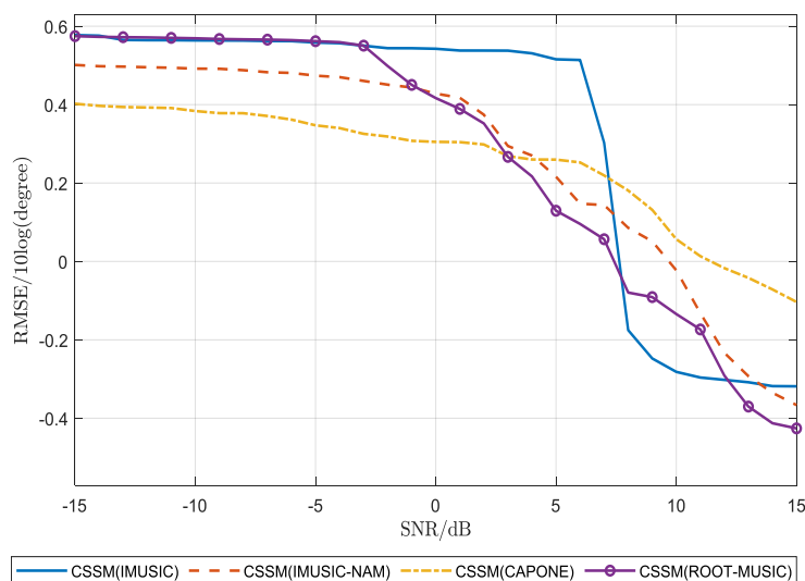
Рис. 5. Графіки залежностей СКВ оцінок алгоритму CSSM від ВСШ при первинній обробці сигналу з використанням алгоритмів IMUSIC, IMUSIC-NAM, CAPONE, ROOT-MUSIC
