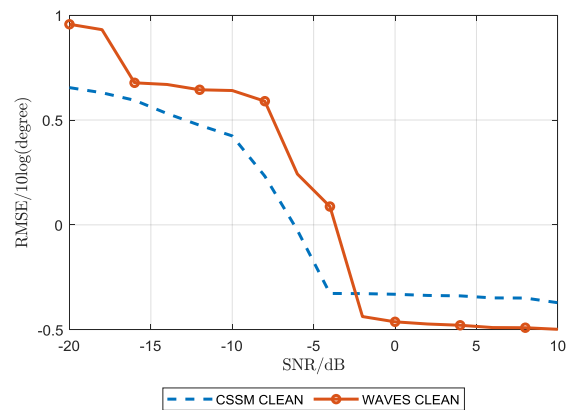
Рис. 8. Графики залежностей СКВ оцінок алгоритмів CSSM-CLEAN, WAVES-CLEAN від ВСШ
