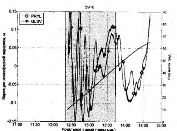
Рис. 6. Вариационные составляющие ионосферной задержки для различных комбинаций референционных станций и «роверных» пунктов
