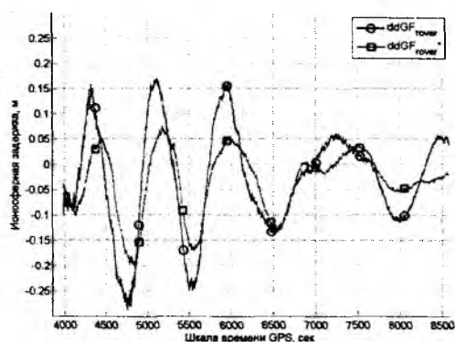
Рис. 7. Исходные и интерполированные двойные разности ионосферных задержек на базе «SHDA»-GLSV: а – для спутников SV18-SV21, б – для спутников SV10-SV21
