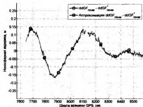
Рис. 14. Двойные разности ионосферных задержек после ввода сетевых коррекций и результаты их полиномиальной аппроксимации (использовались полиномы Лежандра) на базе «BOBR»-GLSV: а – для спутников SV15-SV21, б – для спутников SV22-SV21
