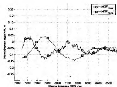
Рис. 12. Двойные разности ионосферных задержек после ввода сетевых коррекций и результаты их полиномиальной аппроксимации (использовались полиномы Лежандра) на базе «BOBR»-GLSV: a – для спутников SV18-SV21, б – для спутников SV22-SV21
