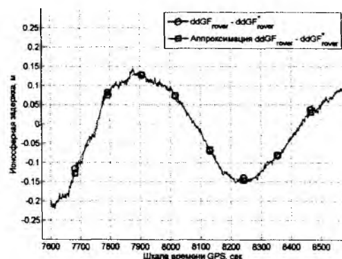
Рис. 9. Исходные и интерполированные двойные разности ионосферных задержек на базе «SHDA»-GLSV: a – для спутников SV15-SV21, б – для спутников SV22-SV21
