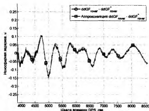
Рис. 11. Исходные и экстраполированные двойные разности ионосферных задержек на базе «BOBR»-GLSV: a – для спутников SV18-SV21, б – для спутников SV10-SV21
