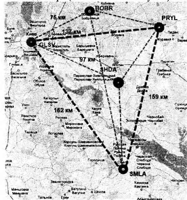
Рис. 3. Карта расположения референционных станций и роверных приемников потребителей
