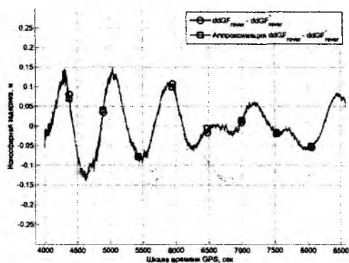
Рис. 8. Двойные разности ионосферных задержек после ввода сетевых коррекций и результаты их полиномиальной аппроксимации (использовались полиномы Лежандра) на базе «SHDA»-GLSV: a – для спутников SV18-SV21, б – для спутников SV10-SV21
