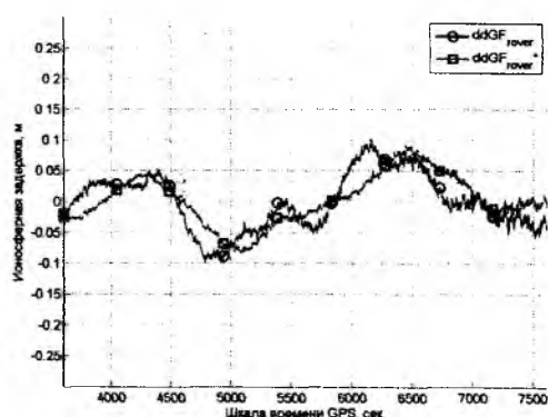
Рис. 7. Исходные и интерполированные двойные разности ионосферных задержек на базе «SHDA»-GLSV: а – для спутников SV18-SV21, б – для спутников SV10-SV21
