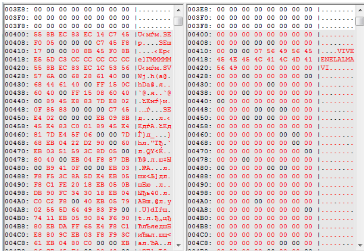
Рисунок 4.7 – Порівняння копій NrgBot
