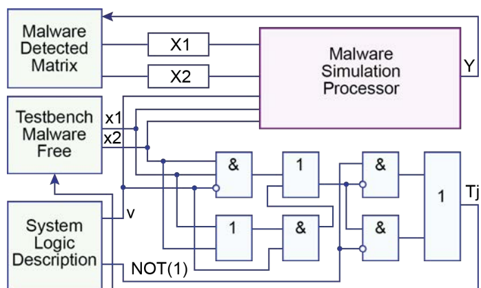
Рисунок 2.9 – HFS-структура апаратного моделювання
