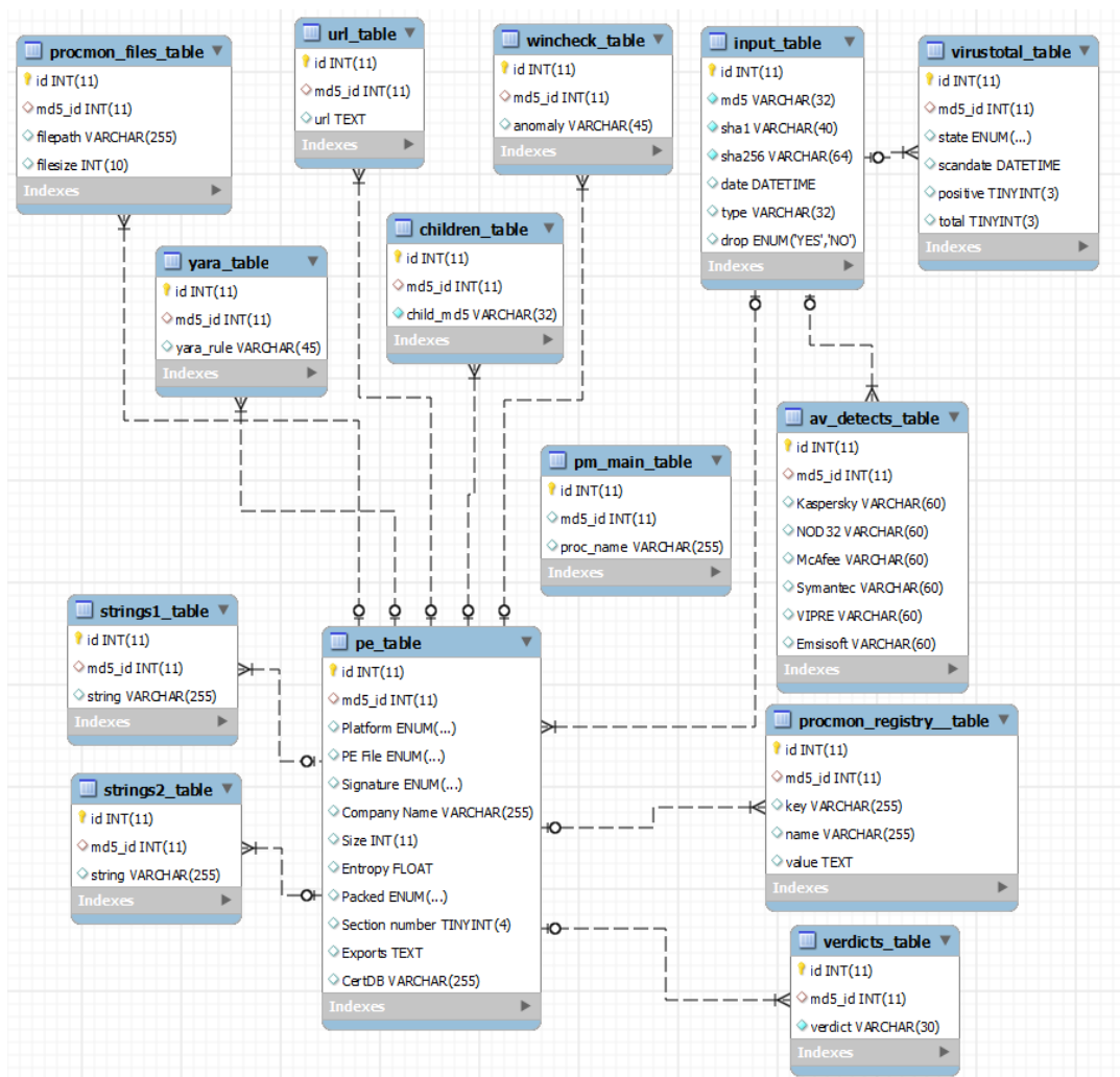
Рисунок 5.2 – Database Architecture
