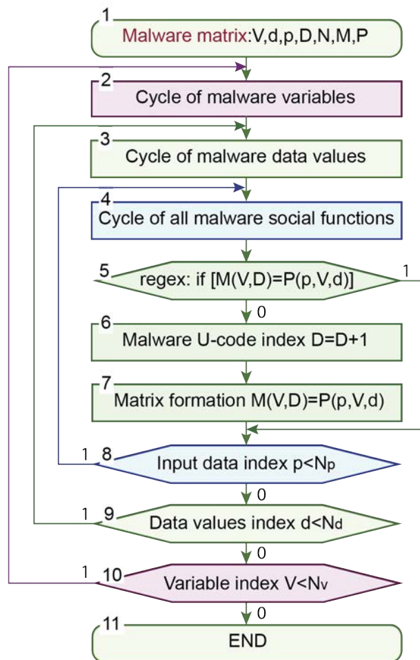
Рисунок 3.10 – Алгоритм формування матриці значень параметрів
