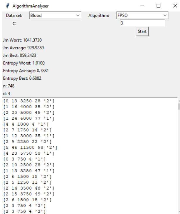
Рисунок А.2 – Результат роботи FPSO алгоритму
