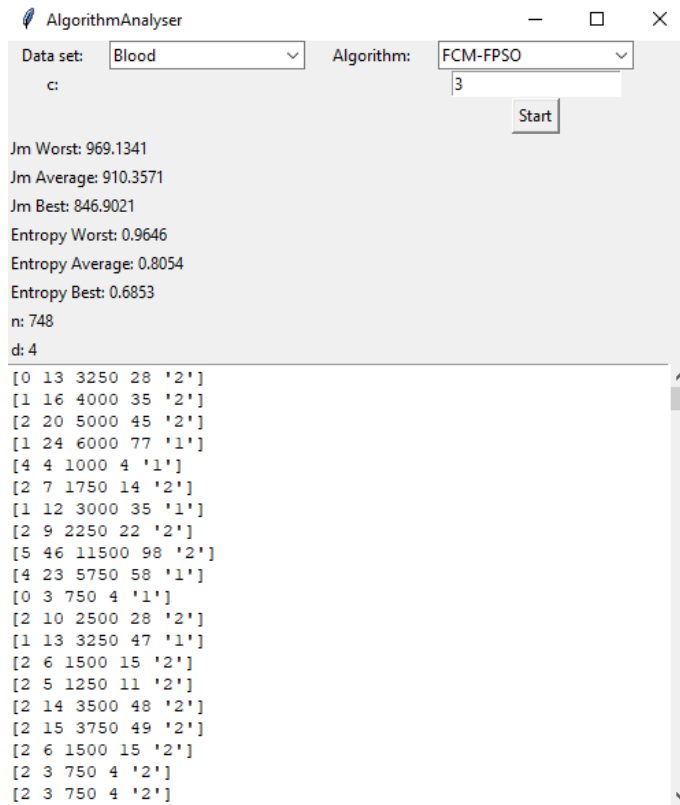
Рисунок А.3 – Результат роботи FCM-FPSO алгоритму
