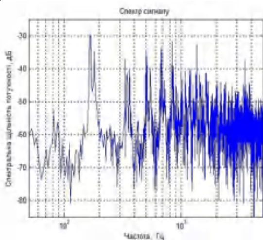
Рисунок 1 - Спектр АВ квадрокоптера DJI Phantom 3T
