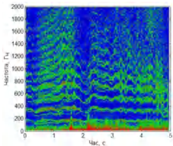
Рисунок 2 - Спектрограма складових АВ квадрокоптера DJI Phantom 3T
