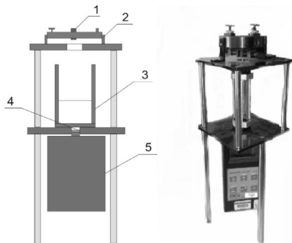
Рисунок 3 – Схема виміральної установки для вимірювання коефіцієнту поглинання води: 1 – коліматор Thorlabs 260с-FC; 2 – юстирувальний вузол; 3 – кювета; 4 – світлофільтр; 5 – оптичний тестер EXFO FOT-90
