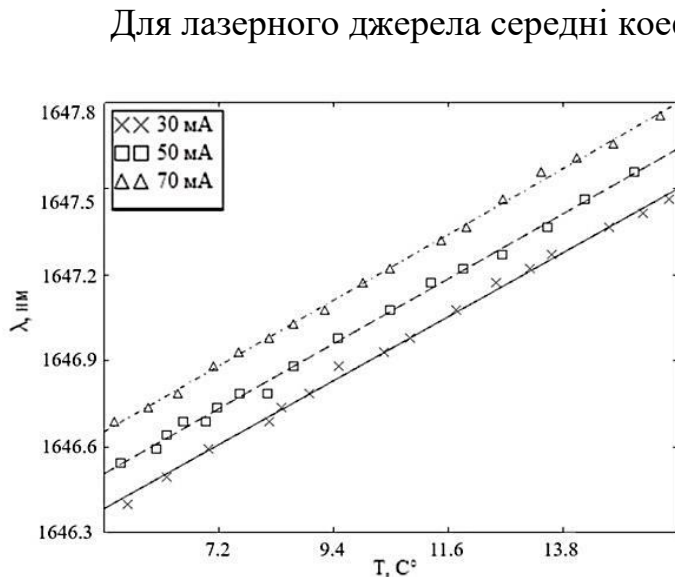
Рисунок 7 – температурна перебудова довжини хвилі лазерного діоду з розподіленим зворотнім зв'язком
