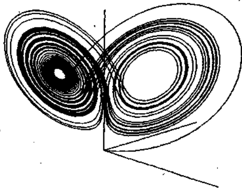
Рис. 3. Поведение решения в фазовом пространстве при наличии странных аттракторах
