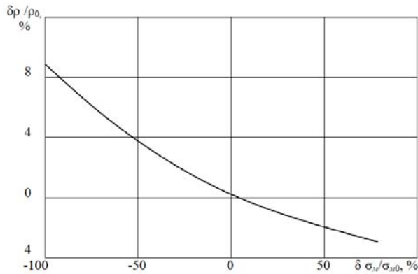
Рис.7. Відносні збільшення величини \rho від дії відносного механічного навантаження \delta\sigma_m / \sigma_{m0}
