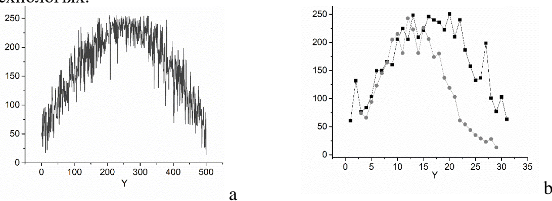
Рис. 1 Моделювання шуму для розподілу інтенсивності у вигляді Гауссова пучка випадковою функцією з коефіцієнтом 0,5 (а). Експериментальний розподіл інтенсивності по осі Y показано сірими колами, а теоретичні розрахунки для цих же точок позначені чорними квадратами.
