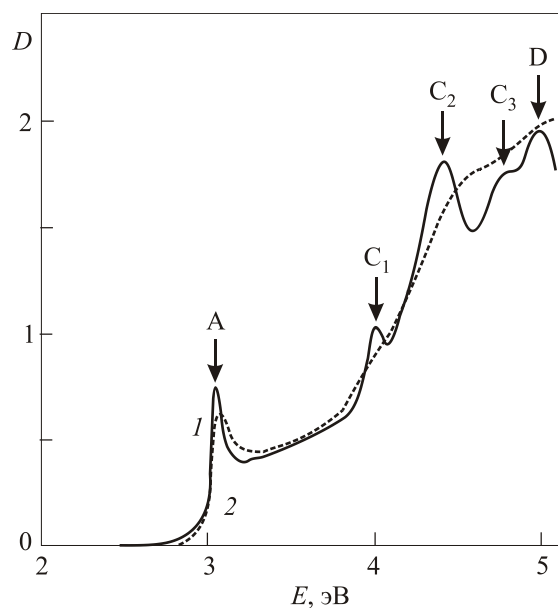
Рис. 1. Спектр поглощения тонкой пленки CsPbCl 3 ( t = 130 нм) при 90 (1) и 290 (2) К.
