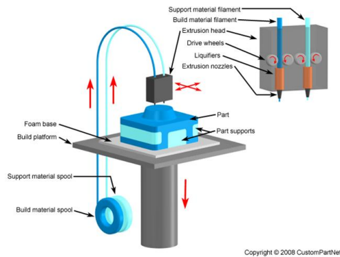
Рисунок 1 –Схема роботи 3D принтерів за технологією FDM
