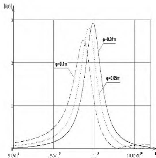
Рис.2. Зависимость АЧХ АРБВ от сдвига фазы сигнала в усилителе
