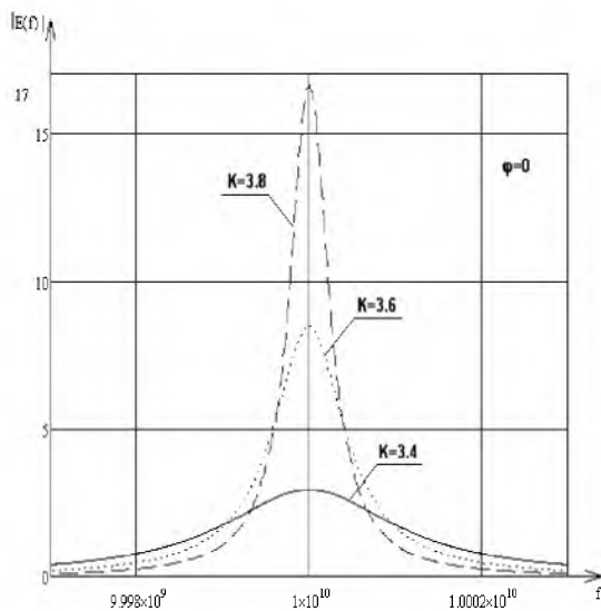
Рис.1. АЧХ АРБВ с нерезонансным усилителем
