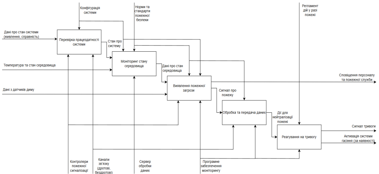
Рисунок 3 – Декомпозиція IDEF0
