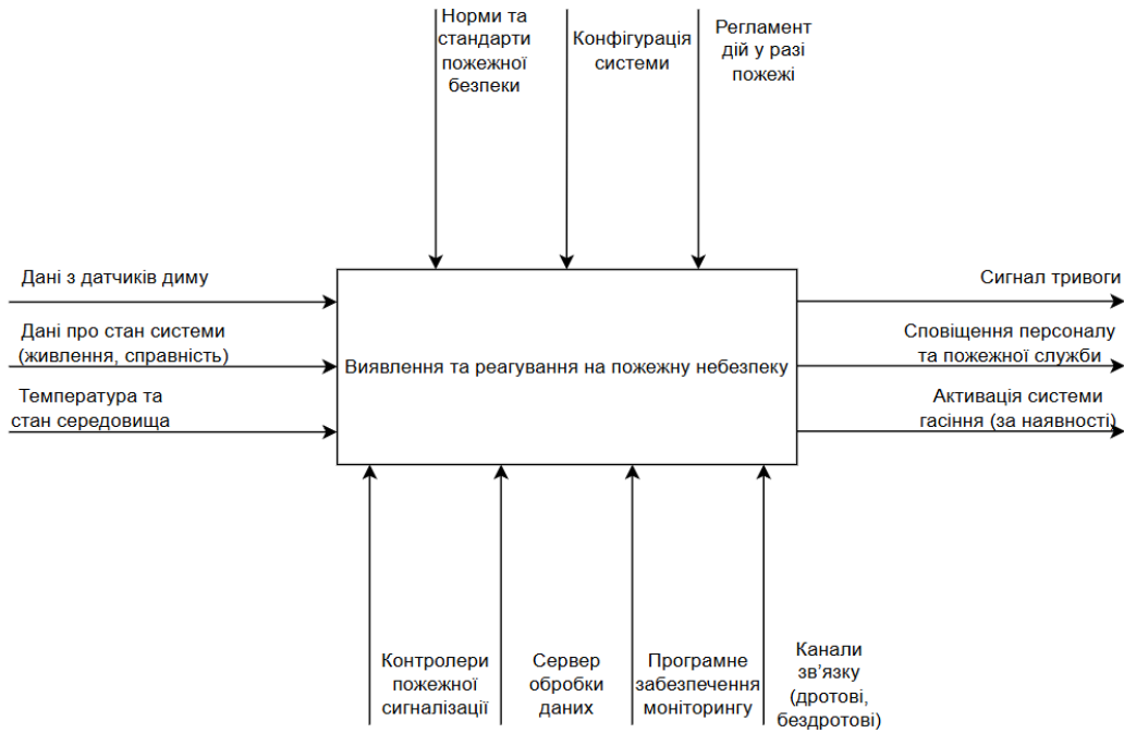
Рисунок 2 – Діаграма IDEF0
