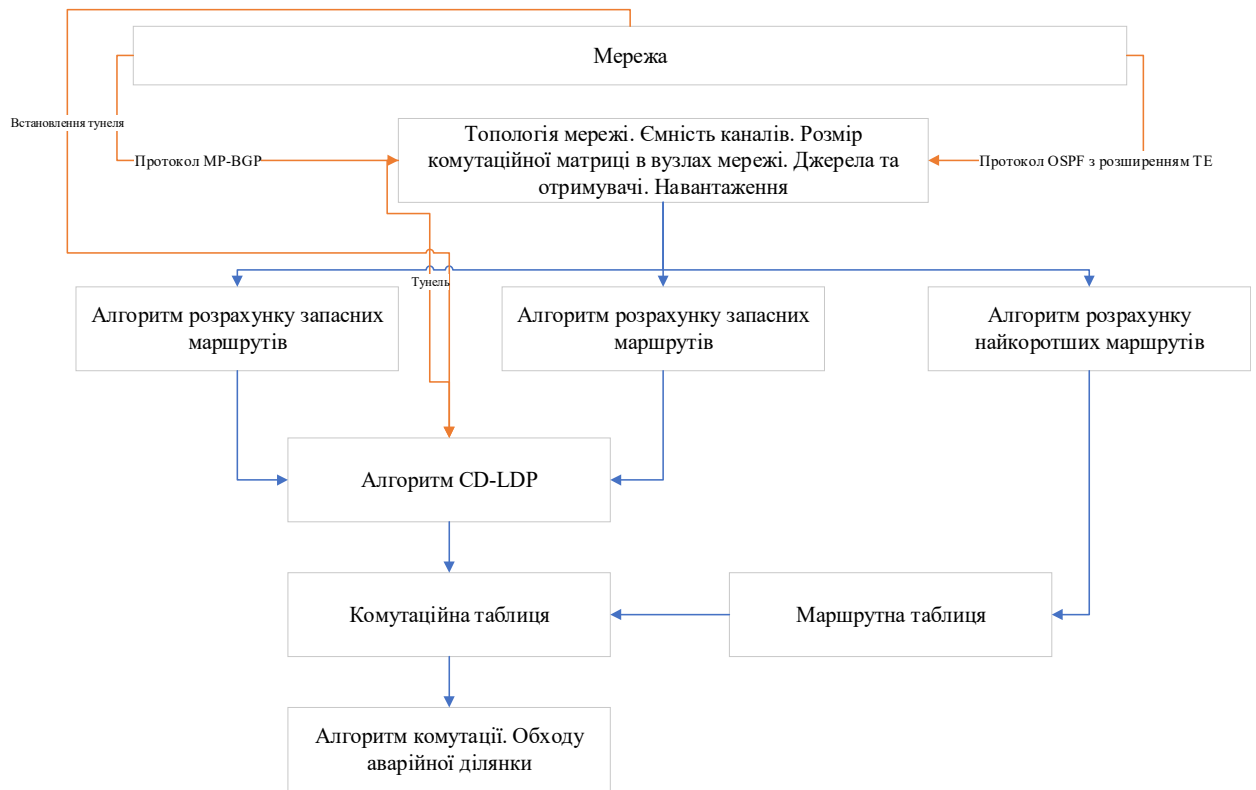
Рисунок 3.6 – Функціональна схема модифікації алгоритму динамічної маршрутизації
