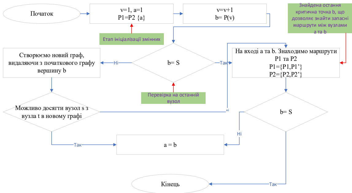
Рисунок 3.4 – Модифікація алгоритму пошуку запасних маршрутів
