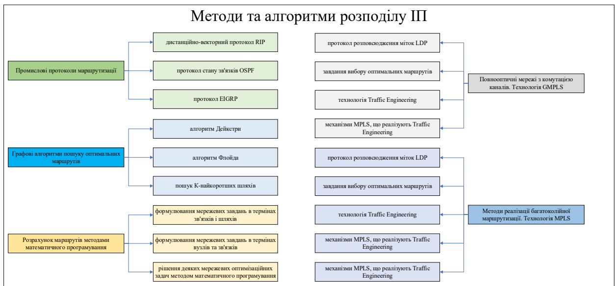
Рисунок 1.9 – Методи та алгоритми розподілу ІІІ
