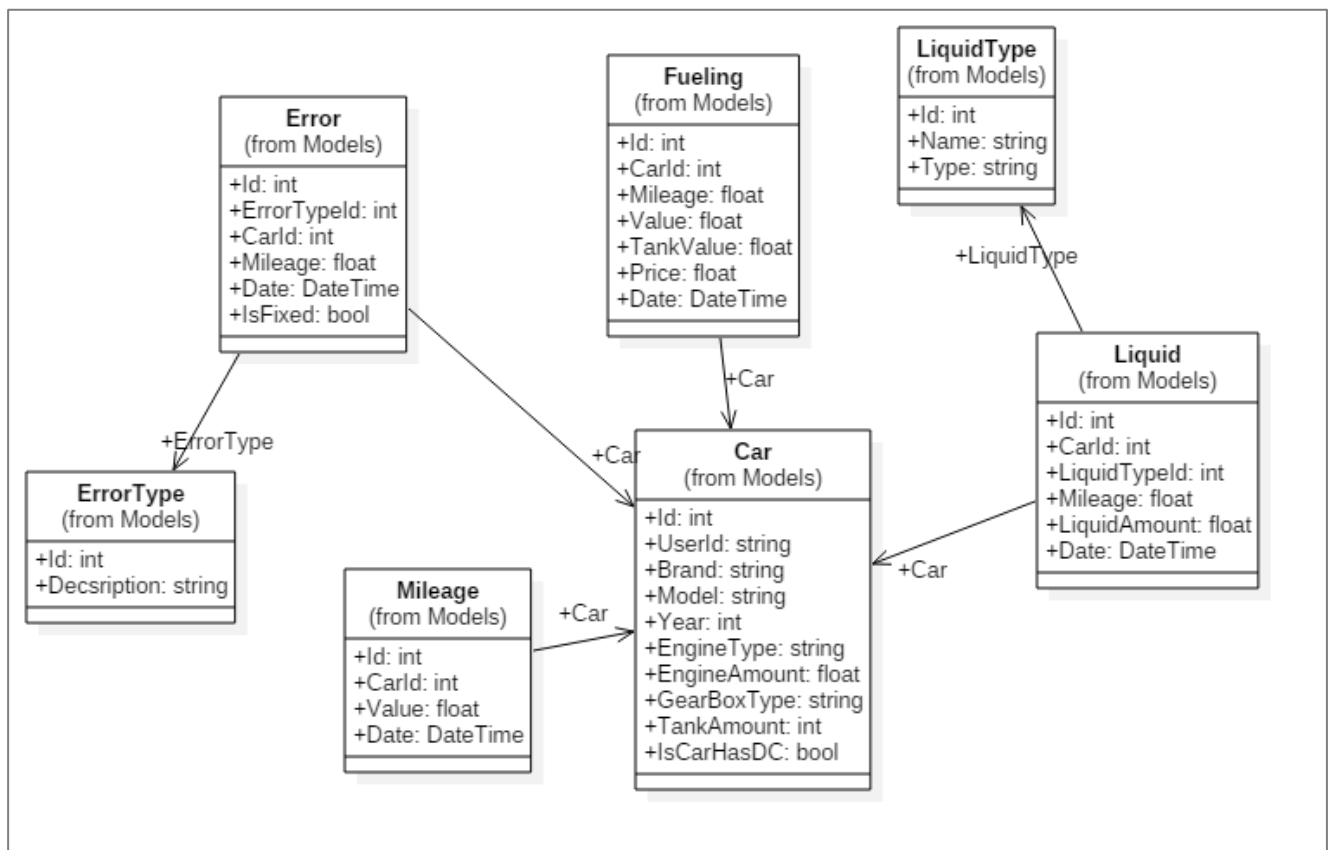
Рисунок 5.2 – Діаграма класів
