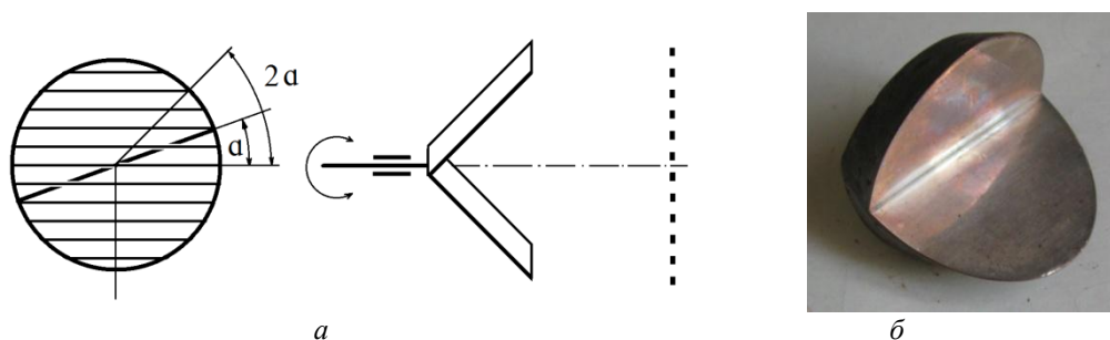
Рис. 1. Схема лазерного резонатора с плавной регулировкой вывода излучения – а ; внешний вид двугранного зеркала – б
