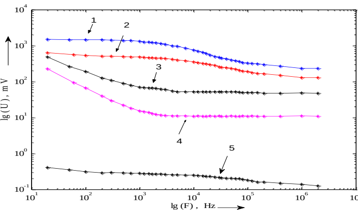
Рис. 3. АЧХ поврежденной клеточной ткани
