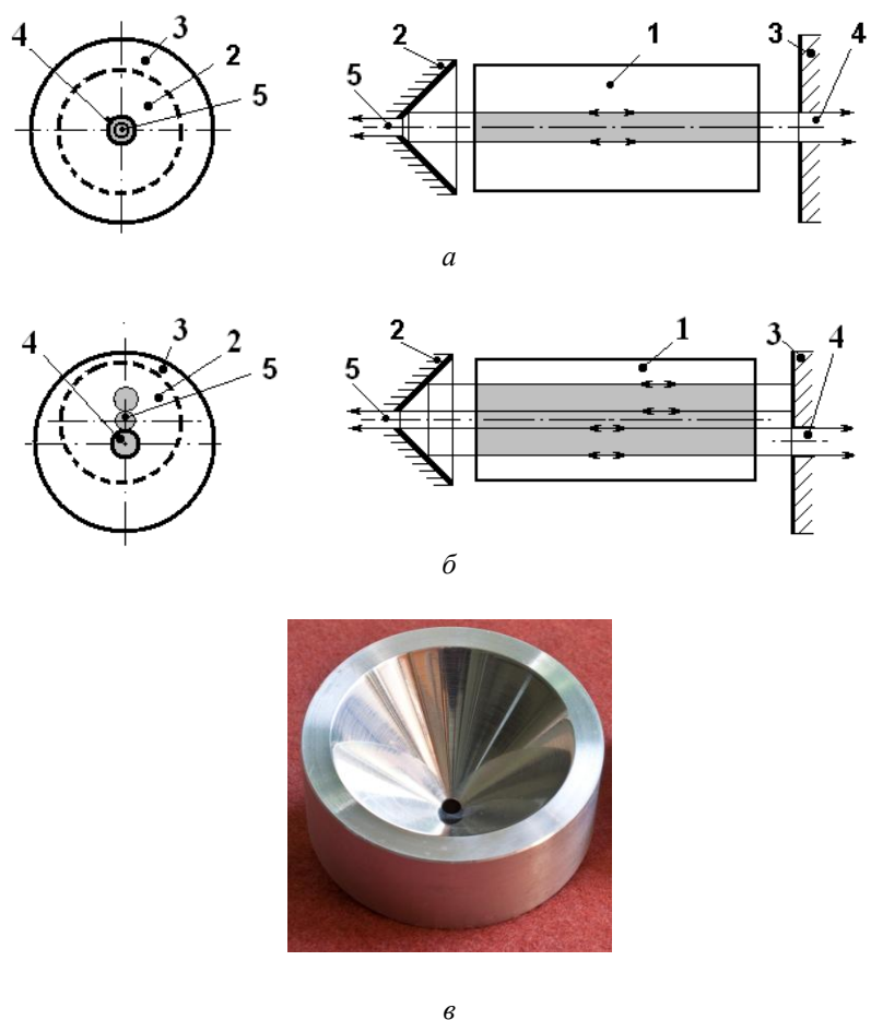
Рис. 4. Схема резонатора с плавной регулировкой, содержащая коническое 90^\circ зеркало с дополнительным каналом не регулируемого вывода излучения (а, б). Внешний вид конического зеркала с отверстием (в)
