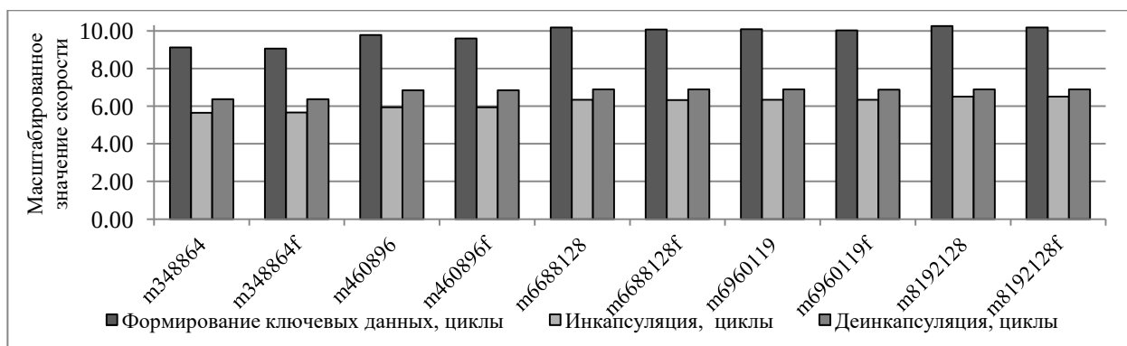
Рис. 9. Гистограмма показателей быстродействия алгоритма Classic McEliece для вычислительной платформы Cortex-A9, в циклах (в логарифмическом масштабе)
