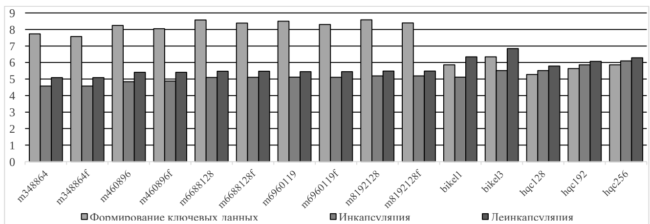
Рис. 8. Гистограмма показателей быстродействия алгоритмов Classic McEliece, BIKE и HQC, в циклах (в логарифмическом масштабе)
