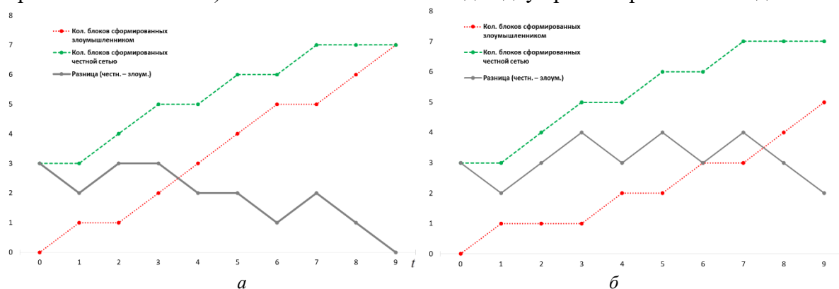
Рис. 1. Пример траектории случайного блуждания: а – для модели независимых игроков; б – для модели разорения игрока
