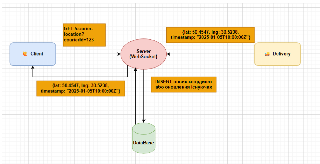
Рисунок А.14 – Схема архітектури головної функції системи
