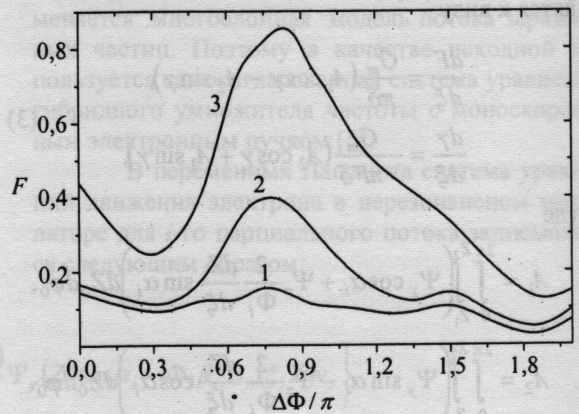
Рис. 3. Зависимости максимальной амплитуды выходного сигнала от параметра расстройки скоростей парциальных потоков, \Phi, b_1 = -3\pi, P_0 = -26 дБ: 1 – I_0/I_{st} = 0,9 ; 2 – 2,5; 3 – 5
