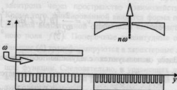
Рис. 1. Схема гибридного умножителя частоты
