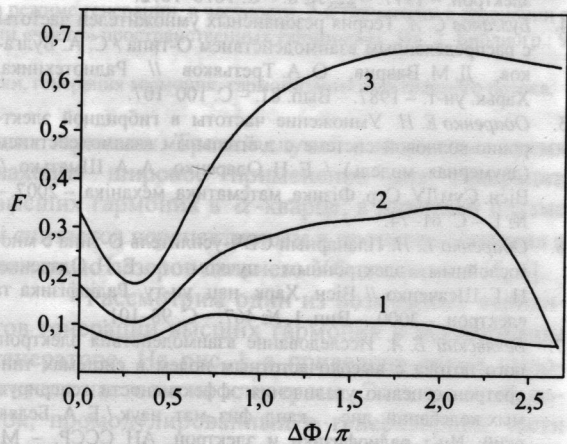
Рис. 8. Зависимости максимальной выходной амплитуды ЛОВ от параметра \Delta\Phi , \Phi_1 b_1 = -\pi/3 , P_0 = -20 дБ: 1 — I_0/I_{st} = 1 ; 2 — 2; 3 — 4
