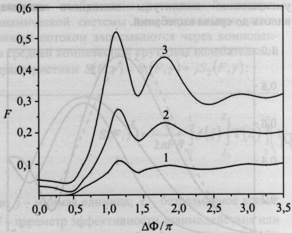
Рис. 5. Зависимости максимальной амплитуды выходного сигнала от параметра \Delta\Phi , \Phi_1 b_1 = -\pi/3 , P_0 = -20 дБ: 1 - I_0/I_{sr} = 0,9 ; 2 - 2,5; 3 - 5
