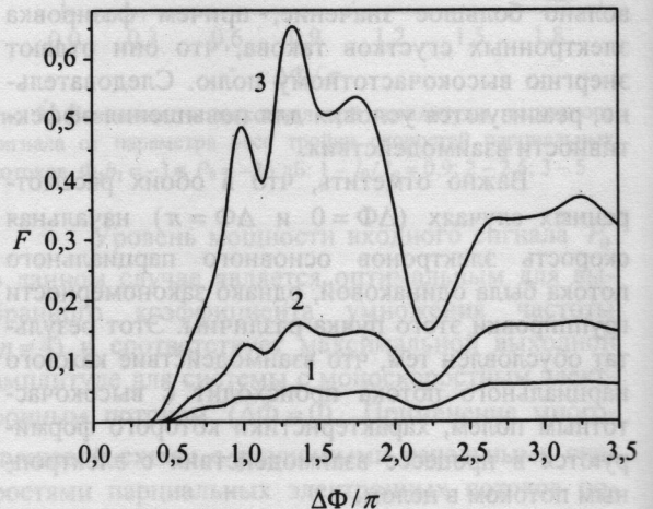
Рис. 7. Зависимости максимальной амплитуды выходного сигнала умножителя от параметра \Delta\Phi , \Phi_1 b_1 = -3\pi , P_0 = -20 дБ: 1 - I_0/I_{sr} = 0,9 ; 2 - 2,5; 3 - 5
