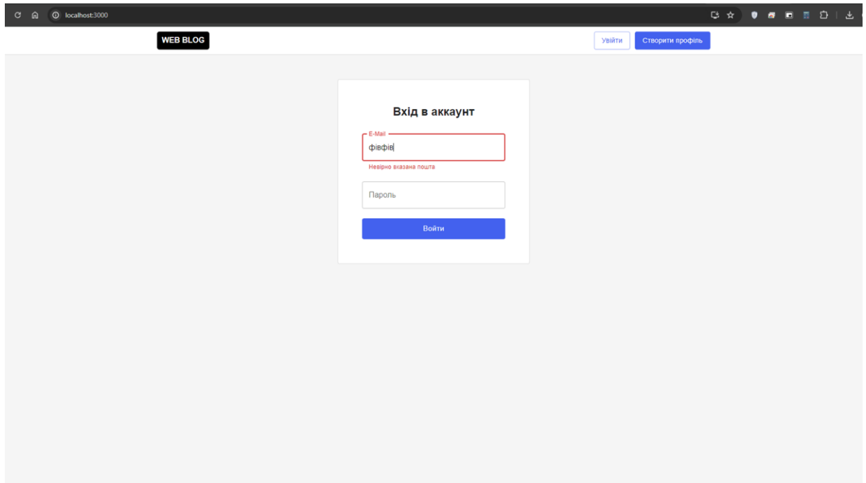
Рисунок 3.2 – Сторінка авторизації
